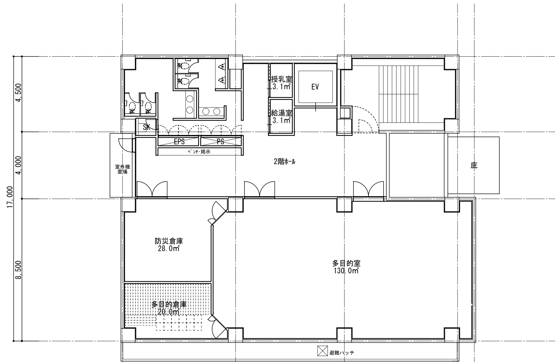
2階平面図
