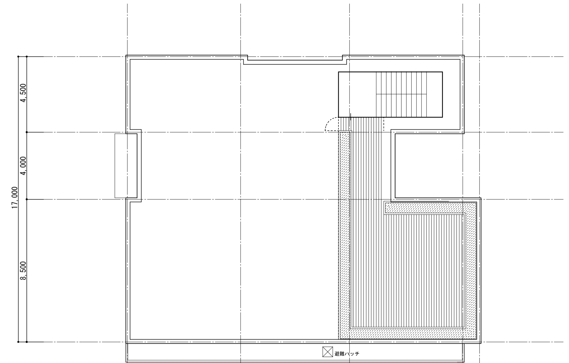
2階平面図
