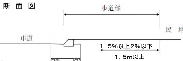
歩道切下げ等に伴う舗装復旧断面図
