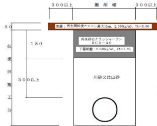
本復旧構造
