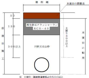
仮復旧構造
