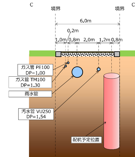
図-2.5 道路内断面図 (C-C' 断面)
