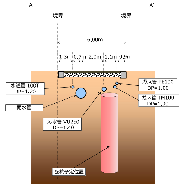
図-2.3 道路内断面図 (A-A' 断面)
