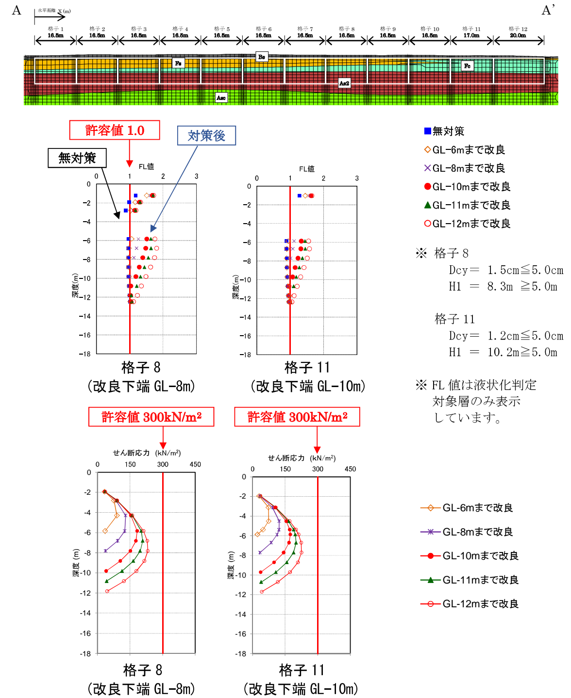
図-2.13 FL値と改良体に発生するせん断応力最大値の深度分布（対策対象地震動 A-A'断面）
