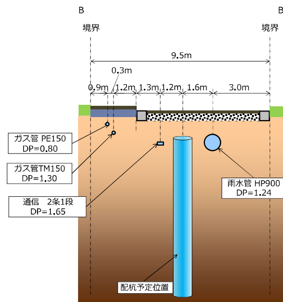
図-2.4 道路内断面図 (B-B' 断面)
