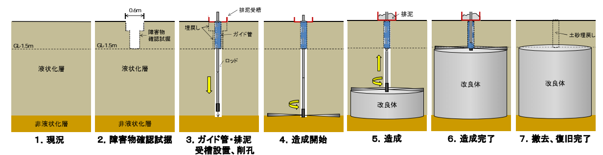
図-2.18 高圧噴射攪拌工法の施工手順 (宅地部を標準)
