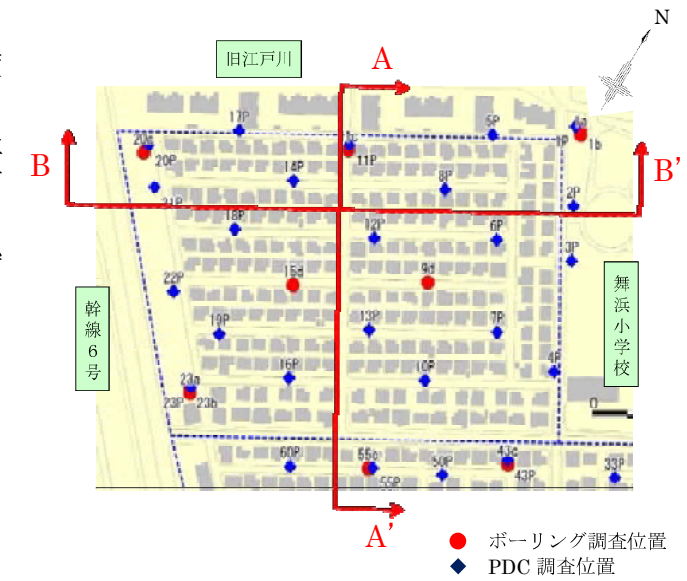
図-1.4 地盤断面位置図
