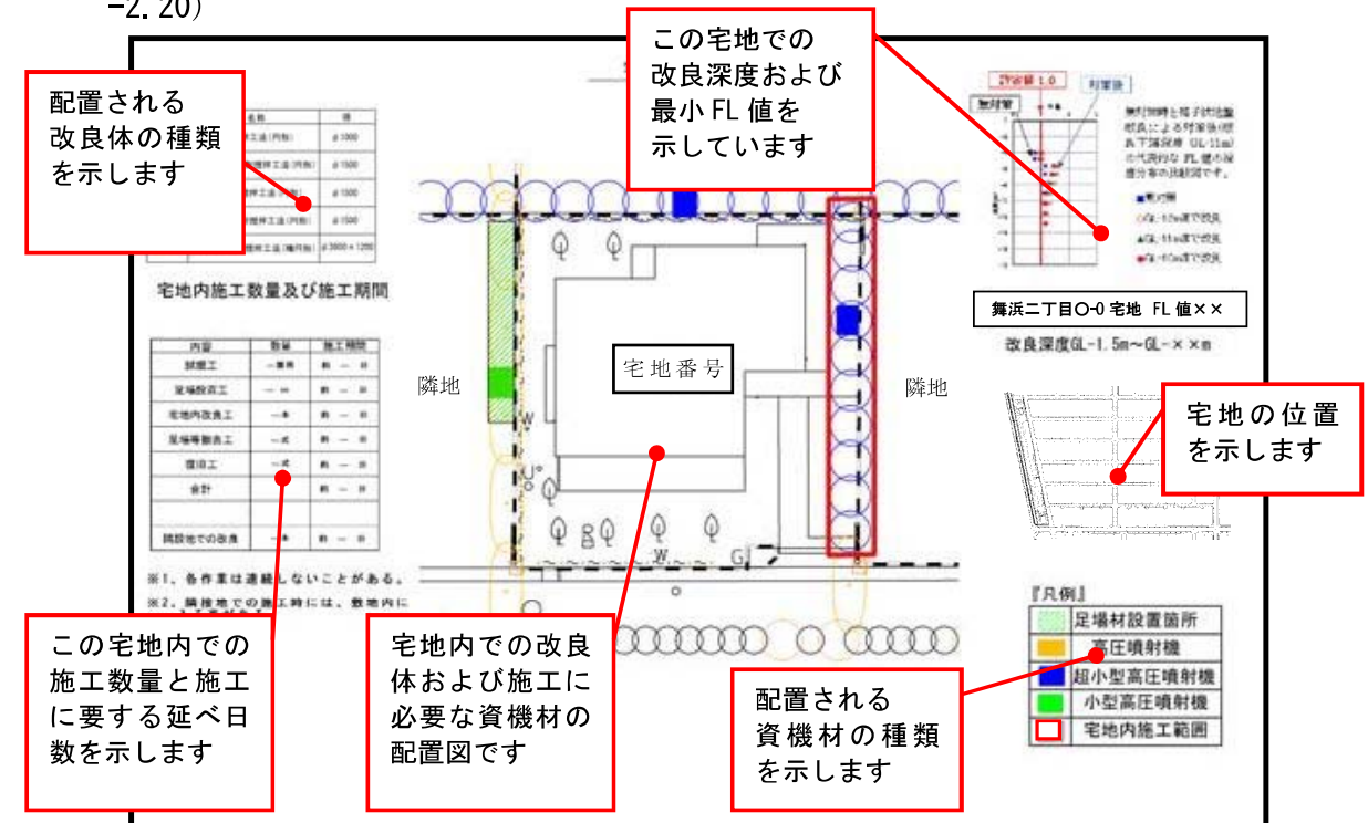
図-2.19 宅地機械配置図の例
