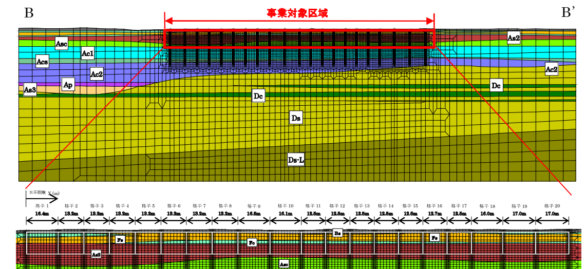
図-2.8 B-B' 断面の擬似3次元解析モデル（上：全体、下：対策範囲拡大）
