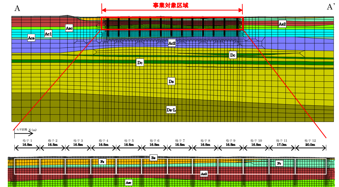
図-2.7 A-A' 断面の擬似3次元解析モデル（上：全体、下：対策範囲拡大）
