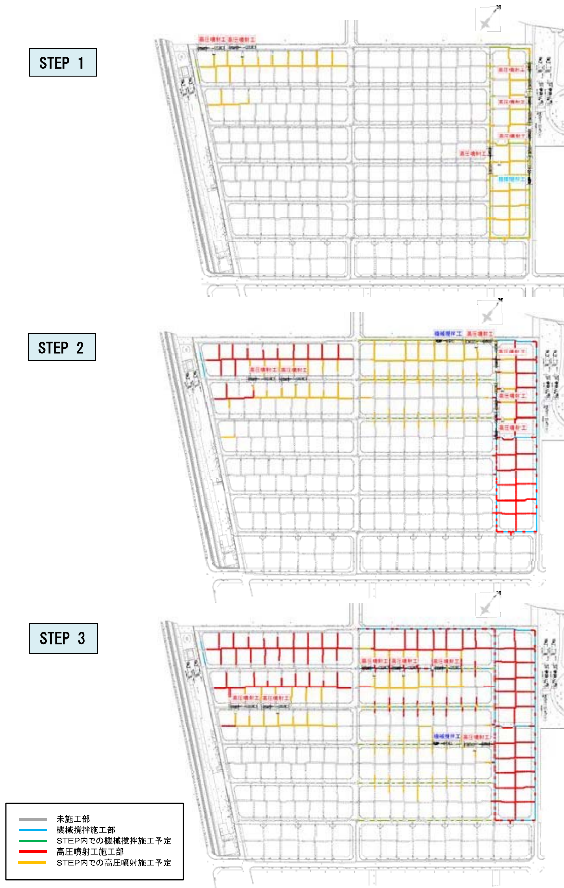
図-2.23 各 STEP における施工状況と機械配置例
