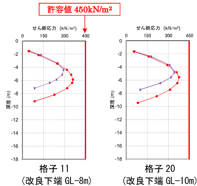
図-2.16 FL 値と改良体に発生するせん断応力最大値の深度分布 (レベル2地震動 B-B' 断面)
