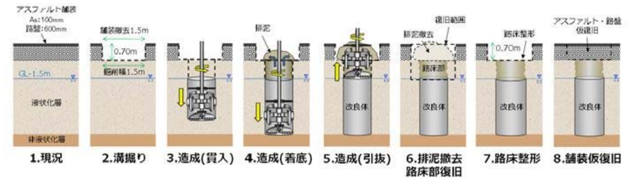
写真-2.1 機械攪拌工法 (円形)
