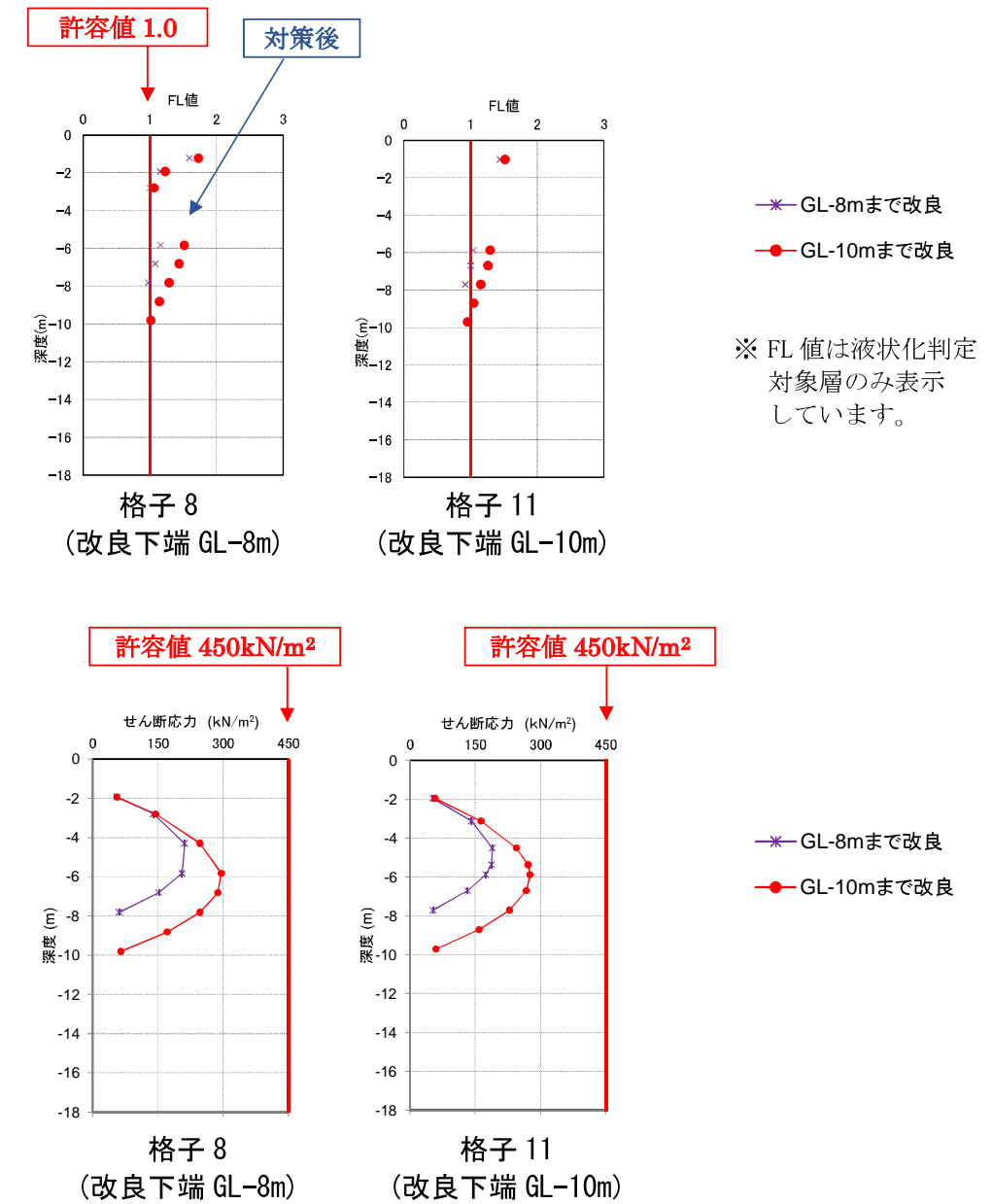
図-2.15 FL 値と改良体に発生するせん断応力最大値の深度分布 (レベル2地震動 A-A' 断面)
