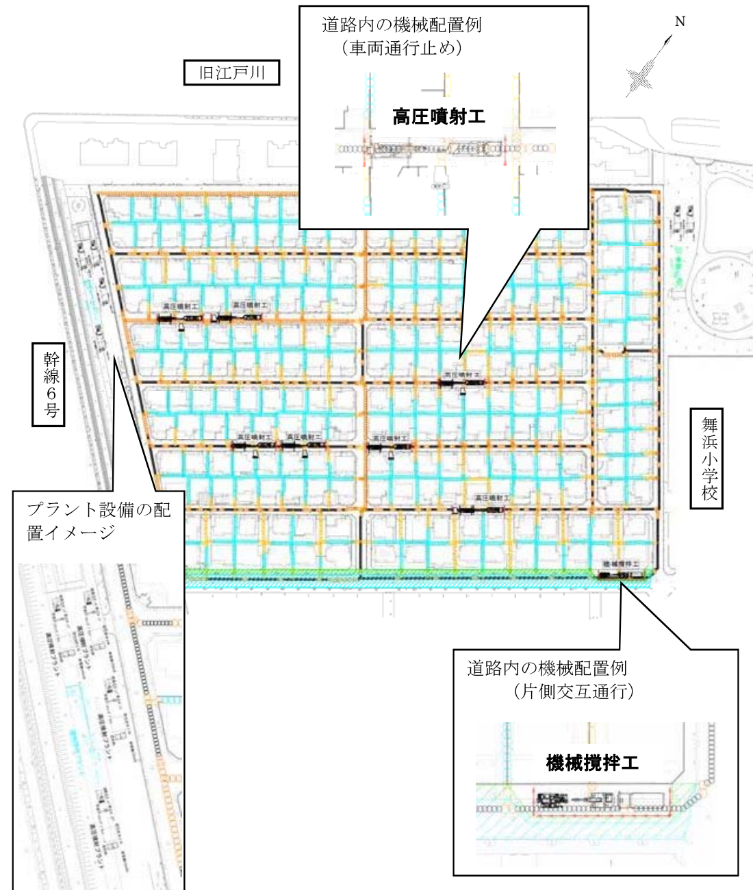
図-2.21 道路および周辺地域での機械配置案
