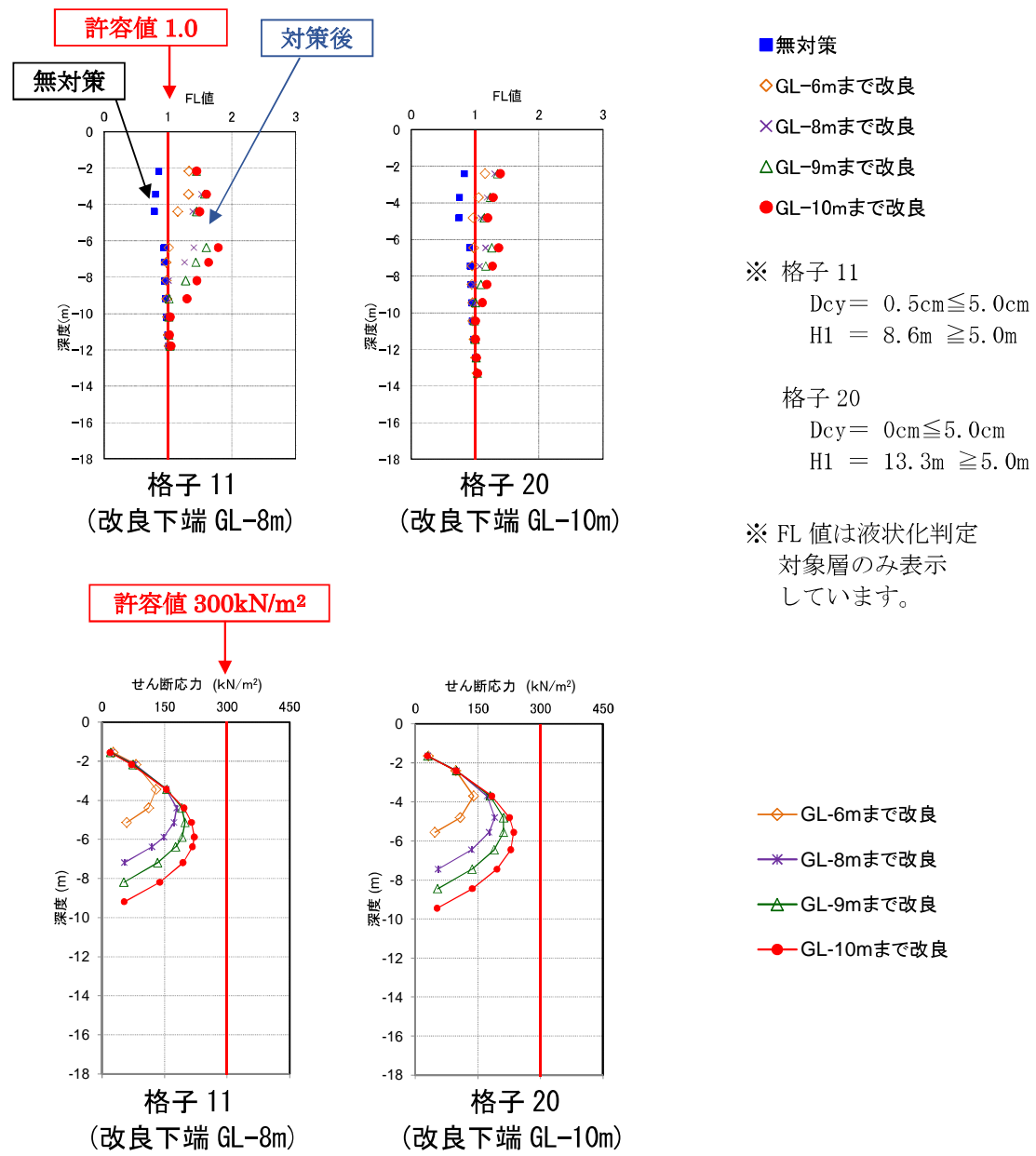
図-2.14 FL 値と改良体に発生するせん断応力最大値の深度分布 (対策対象地震動 B-B' 断面)
