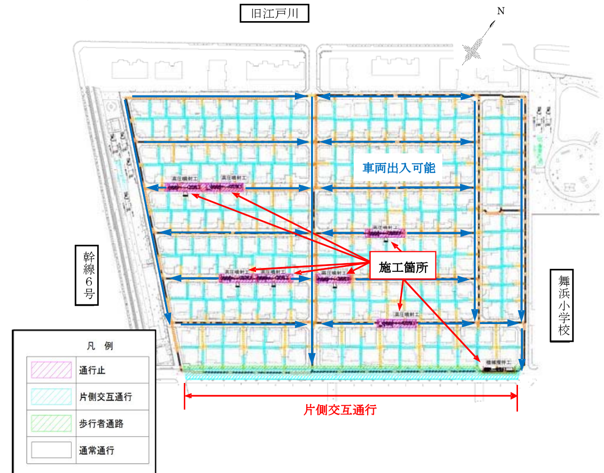
図-2.26 車両通行止めの例（ステップ6のある1日の例）
