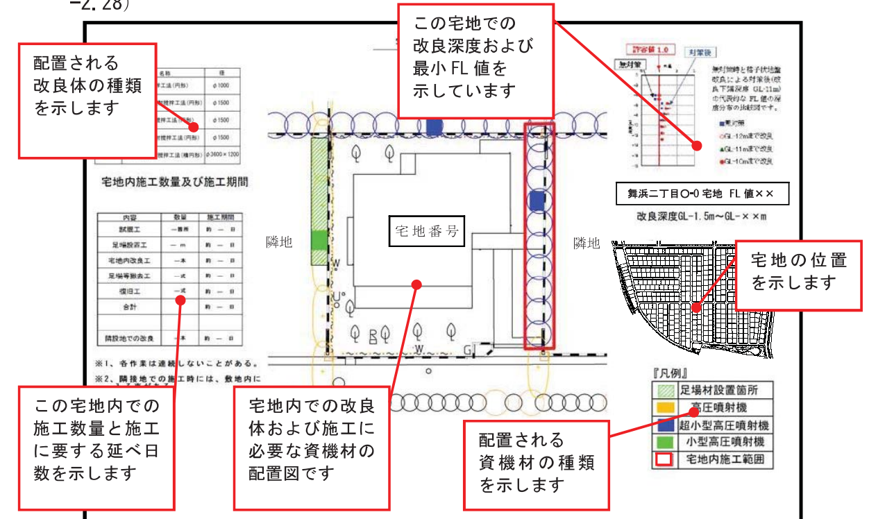
図-2.27 宅地機械配置図の例
