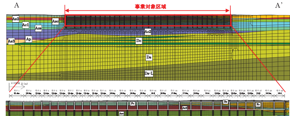
図-2.9 A-A' 断面の擬似3次元解析モデル（上：全体、下：対策範囲拡大）
