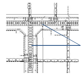
道路覆工板 配置計画例（平面図）
