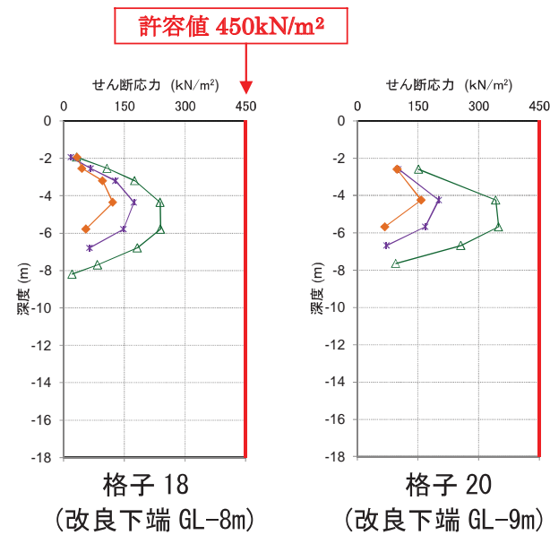
図-2.22 FL 値と改良体が発生するせん断応力最大値の深度分布 (レベル2地震動 B-B' 断面)
