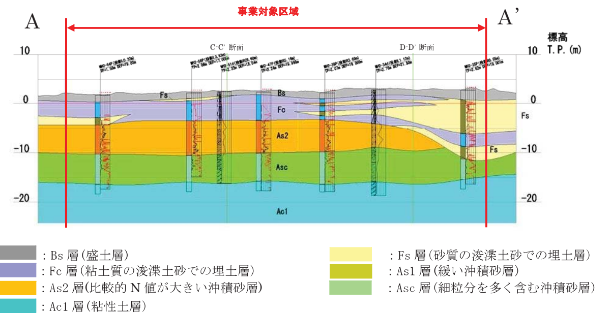
図-1.5 地盤断面図 (1)
