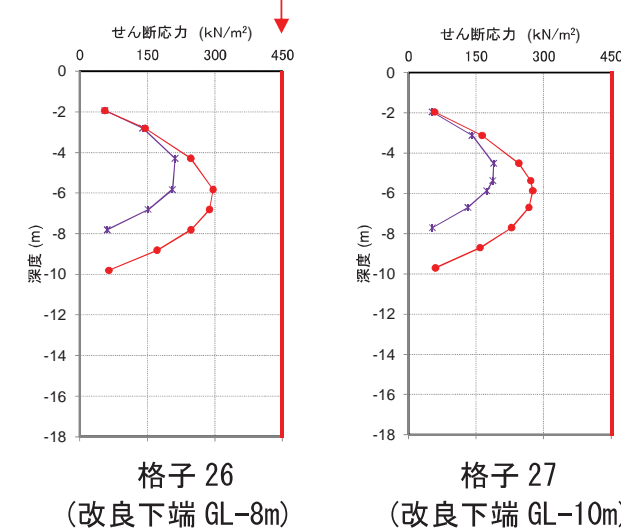
図-2.21 FL 値と改良体に発生するせん断応力最大値の深度分布 (レベル2地震動 A-A' 断面)
