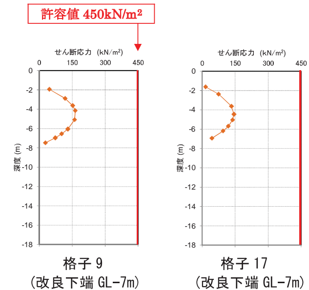
図-2.23 FL 値と改良体が発生するせん断応力最大値の深度分布 (レベル2地震動 C-C' 断面)
