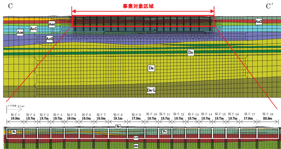
図-2.12 C-C' 断面の擬似3次元解析モデル（上：全体、下：対策範囲拡大）
