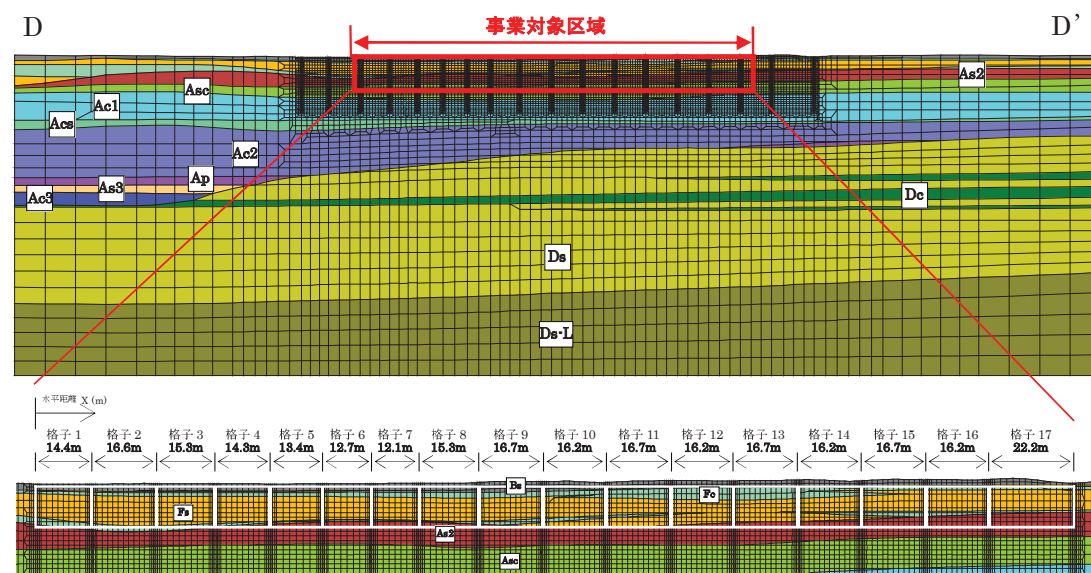
図-2.13 D-D' 断面の擬似3次元解析モデル（上：全体、下：対策範囲拡大）
