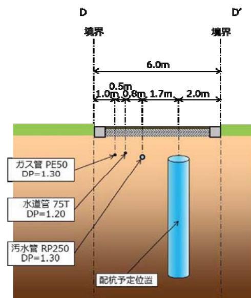
図-2.6 道路内断面図 (D-D' 断面)
