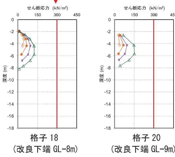
図-2.18 FL 値と改良体が発生するせん断応力最大値の深度分布 (対策対象地震動 B-B' 断面)
