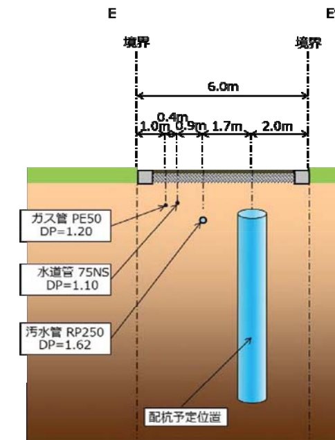
図-2.7 道路内断面図 (E-E' 断面)
