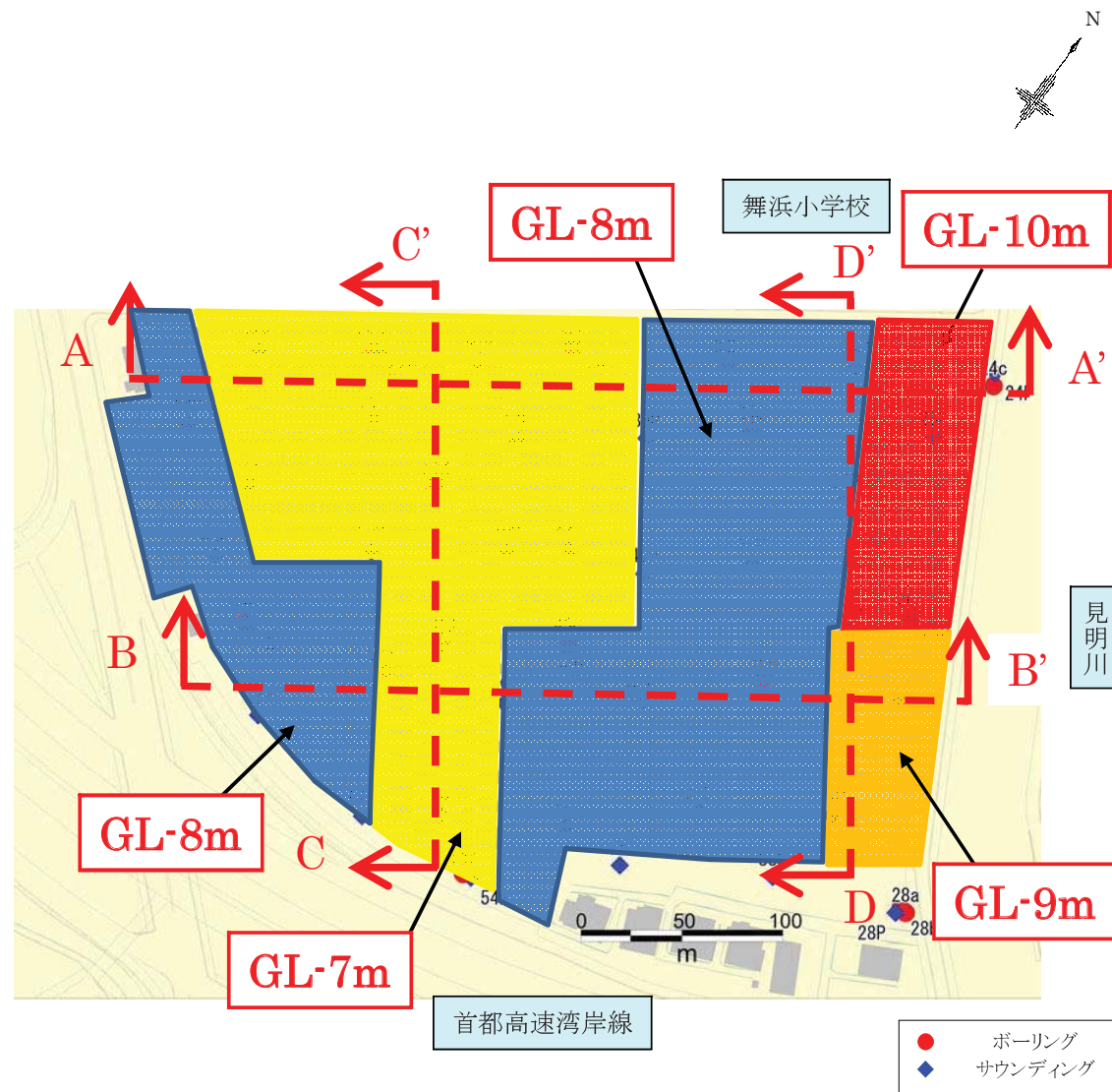
図-2.16 改良体下端深度の平面分布図（舞浜二丁目）
