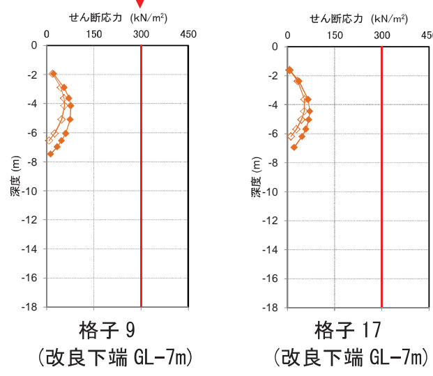
図-2.19 FL 値と改良体が発生するせん断応力最大値の深度分布 (対策対象地震動 C-C' 断面)
