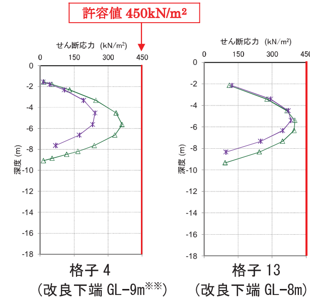
図-2.24 FL値と改良体が発生するせん断応力最大値の深度分布 (レベル2地震動 D-D'断面)
