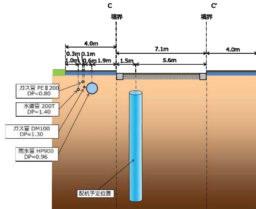
図-2.5 道路内断面図 (C-C' 断面)
