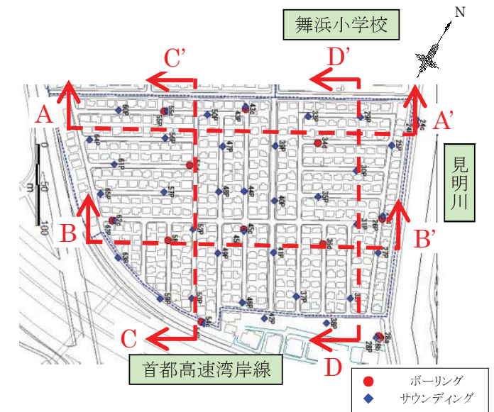
図-1.4 地盤断面位置図
