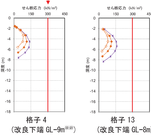
図-2.20 FL 値と改良体に発生するせん断応力最大値の深度分布 (対策対象地震動 D-D' 断面)
