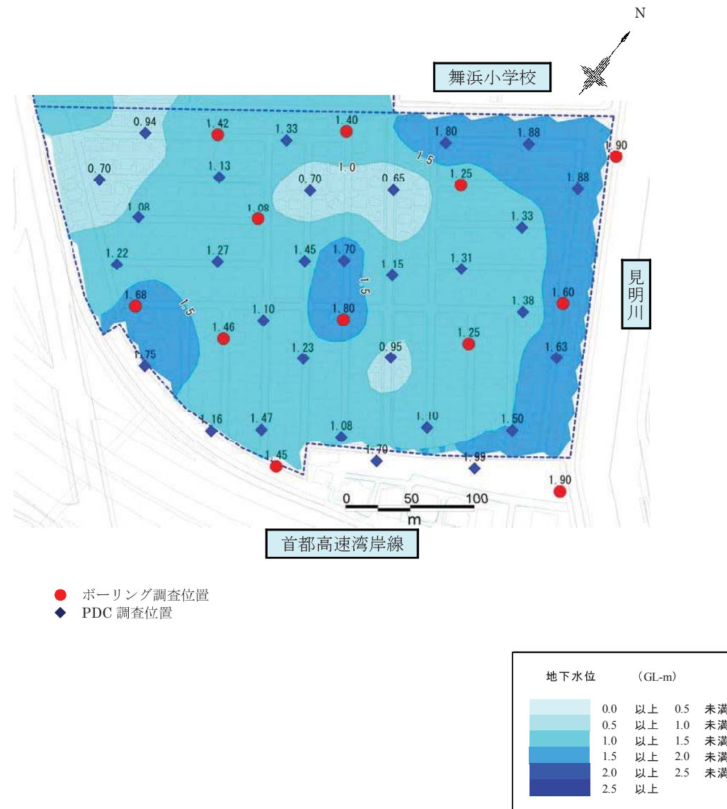
図-1.7 地下水位コンター図
