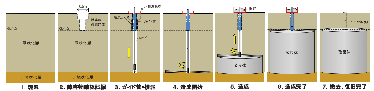
図-2.26 高圧噴射攪拌工法の施工手順 (宅地部を標準)
