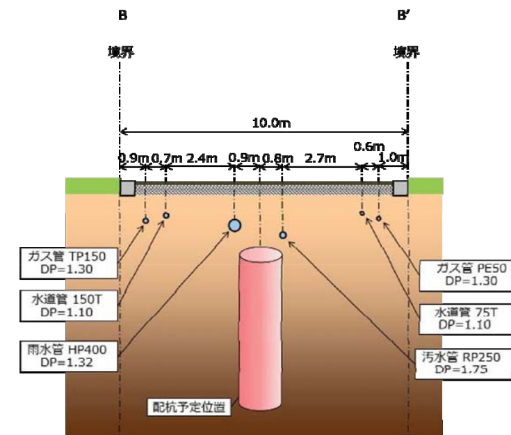
図-2.4 道路内断面図(B-B'断面)
