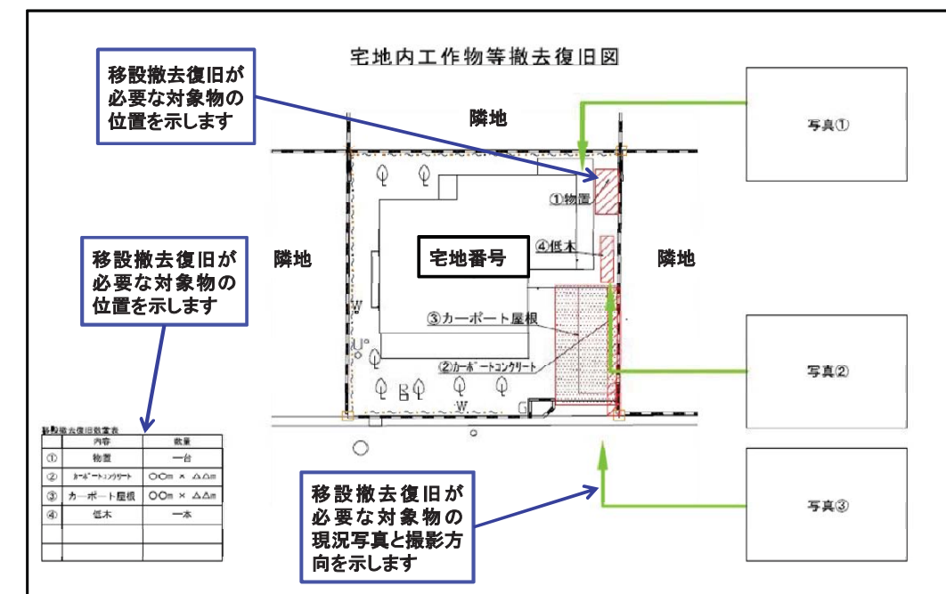
図-2.28 宅地内工作物等撤去復旧図の例
