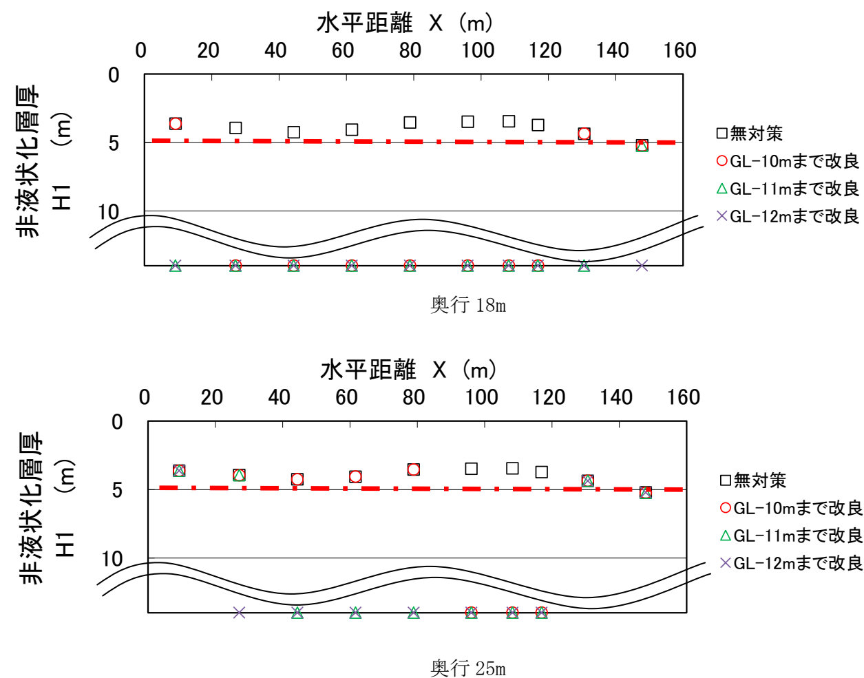
図-11.8 非液状化層厚 H1 の水平分布 (A-A' 断面)
