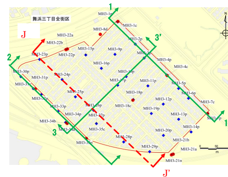
図-13.15 非液状化層厚 H1 の水平分布 (J-J' 断面)
