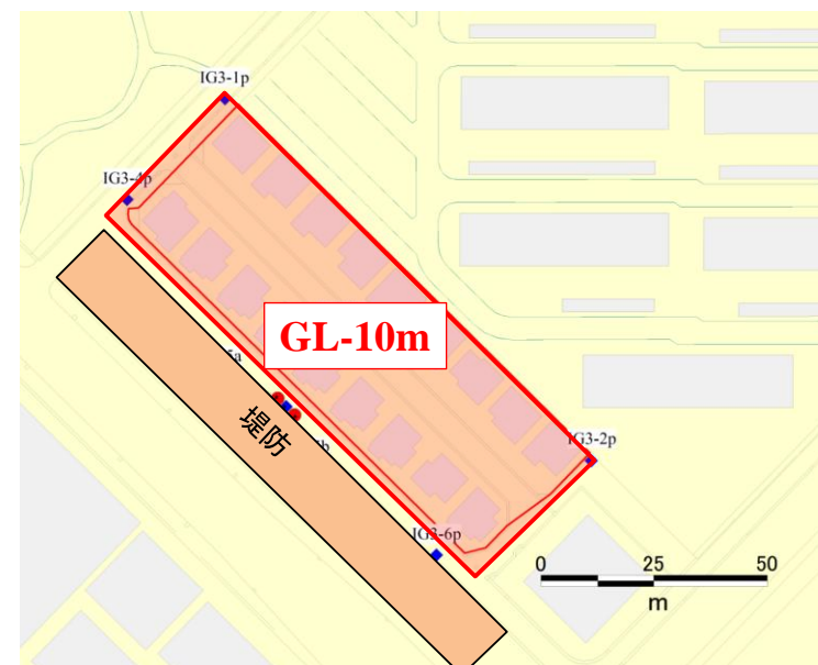
図-10.6 格子状地盤改良下端深度の平面分布図
