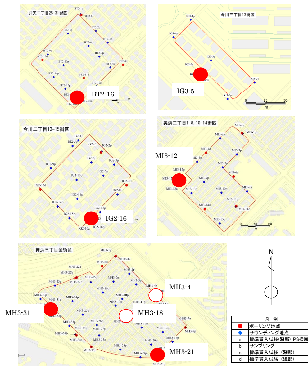
図-8.1 1次元等価線形解析(SHAKE)の実行箇所(図中の赤丸)
