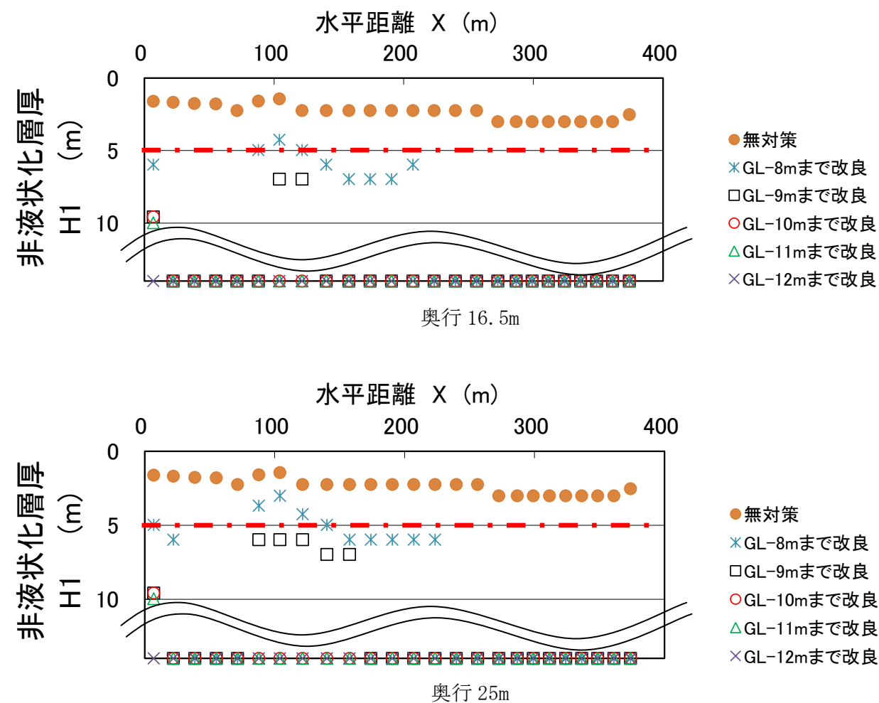
図-13.13 非液状化層厚 H1 の水平分布 (I-I' 断面)
