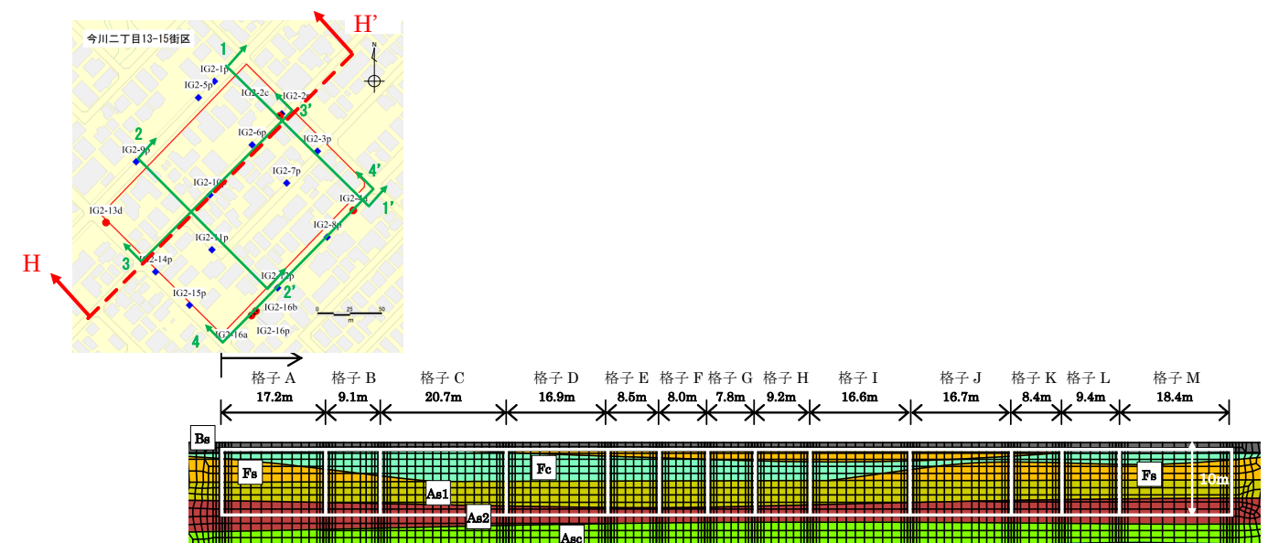
図-14.12 非液状化層厚 H1 の水平分布(H-H' 断面、奥行 15m)
