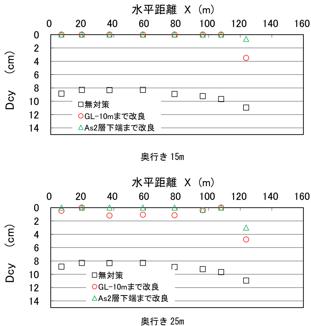
図-14.8 Dcyの水平分布(G-G'断面)
