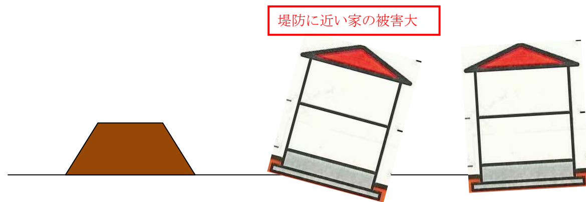
図-10.1 震災時の被害の特徴
