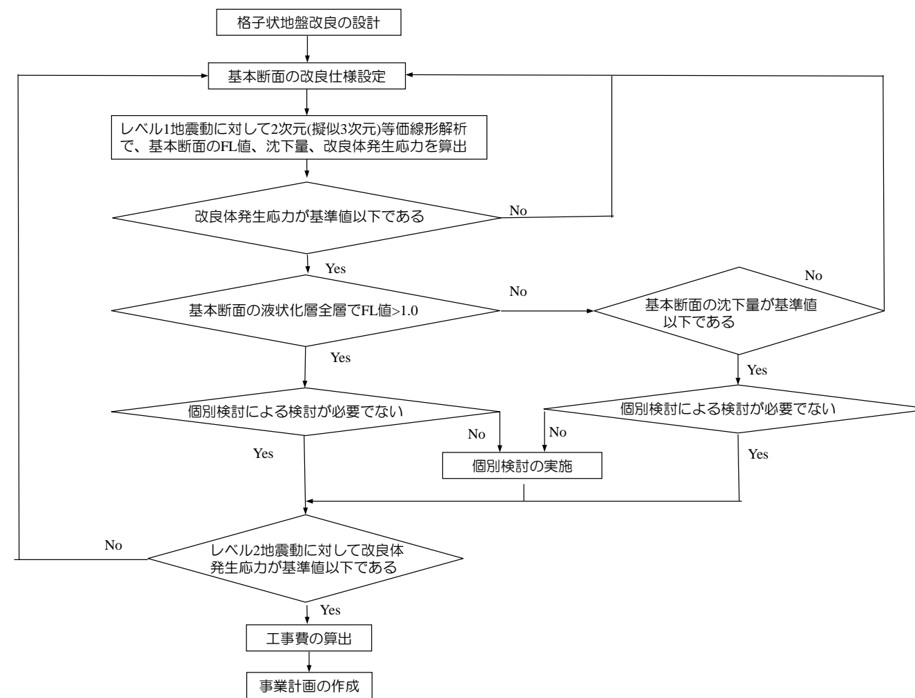
図-6.5 格子状地盤改良工法の設計フロー
