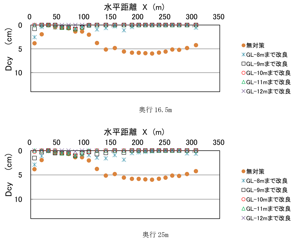
図-13.16 Dcy の水平分布(K-K' 断面)
