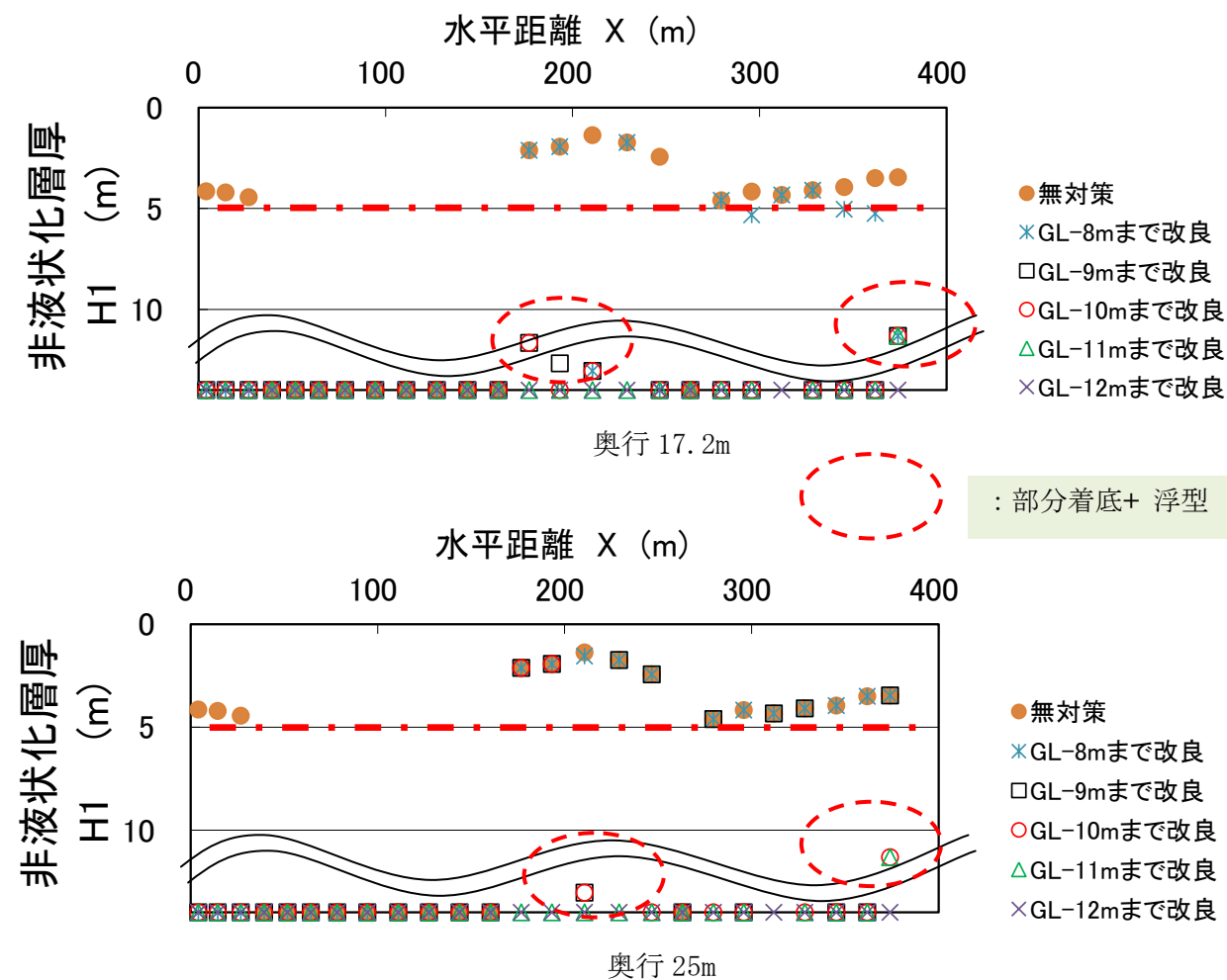
図-13.15 非液状化層厚 H1 の水平分布 (J-J' 断面)
