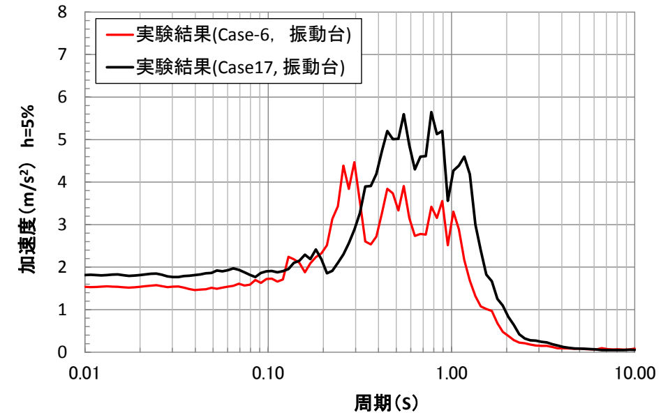
図-5.26 加速度応答スペクトルの比較
