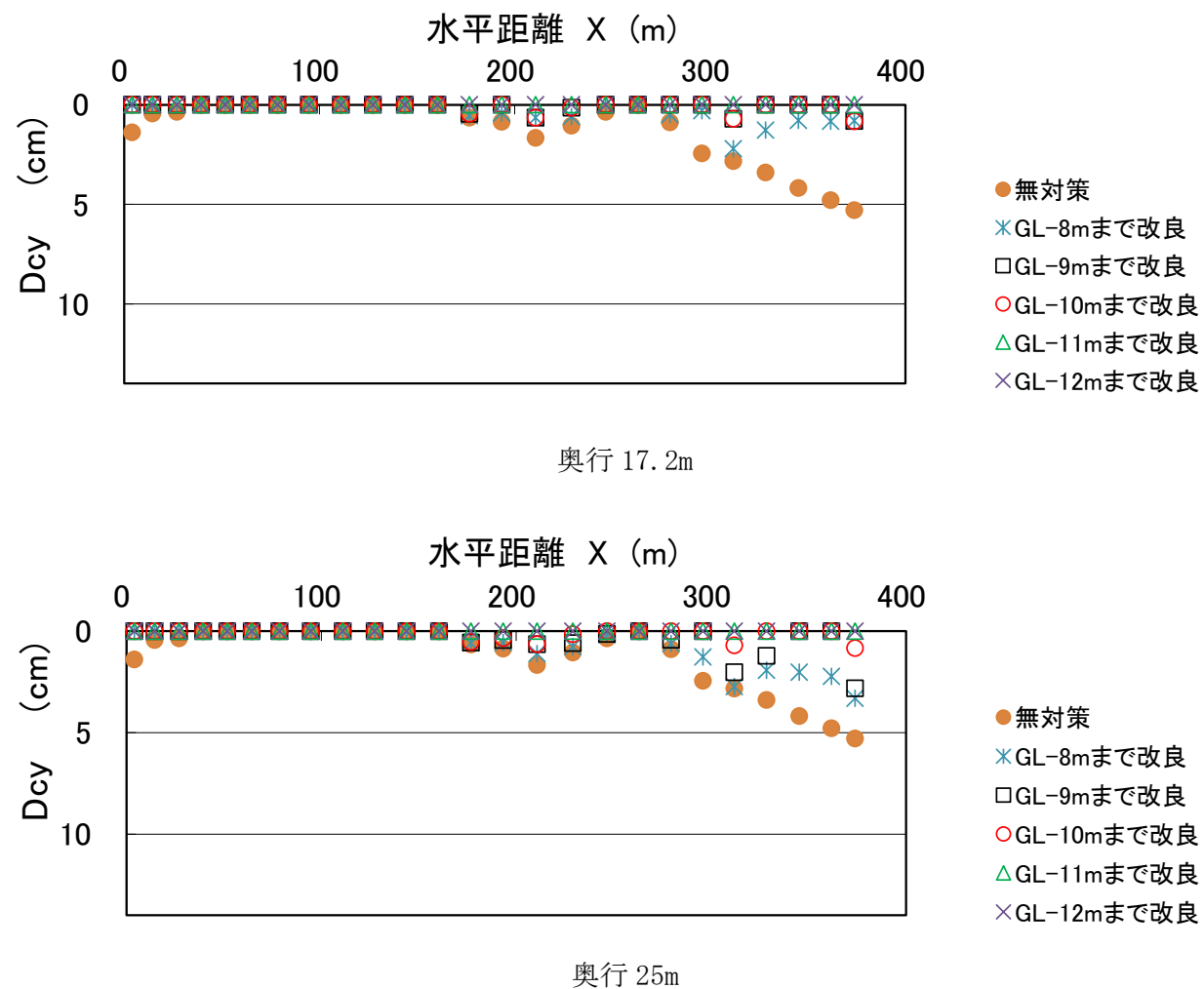
図-13.14 Dcy の水平分布 (J-J' 断面)
