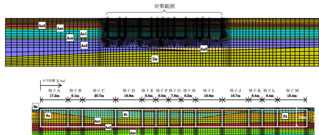
図-14.7 H-H' 断面の解析モデル(上：全体モデル、下：対策範囲を拡大)
