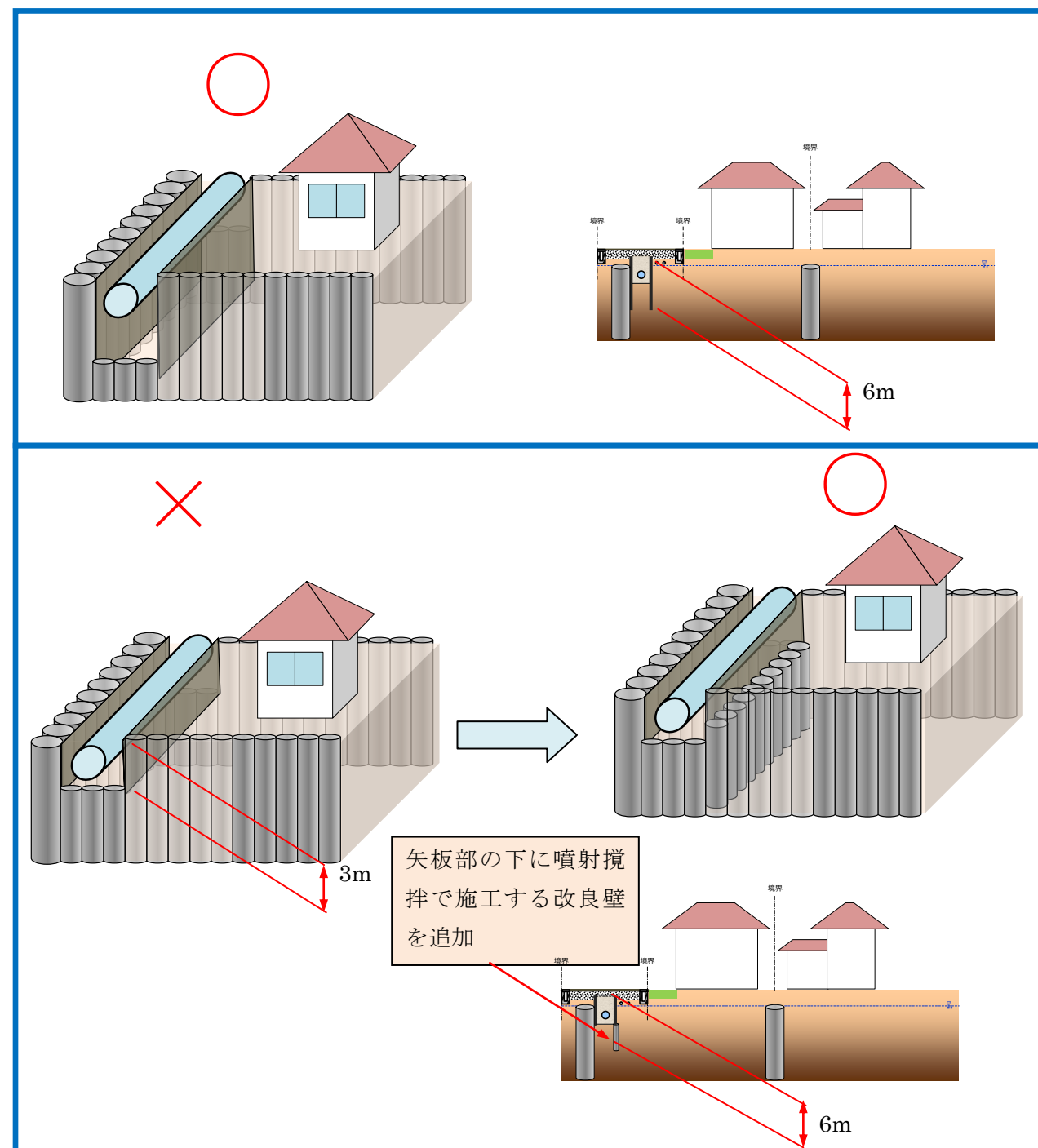
図-5.24 必要な矢板深度(改良壁深度)
