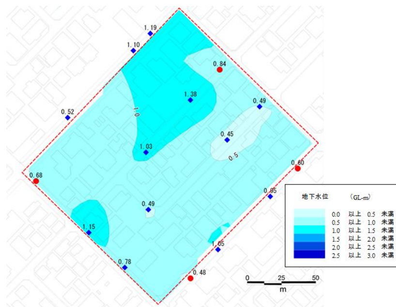
図-14.1 地下水位の計測結果
