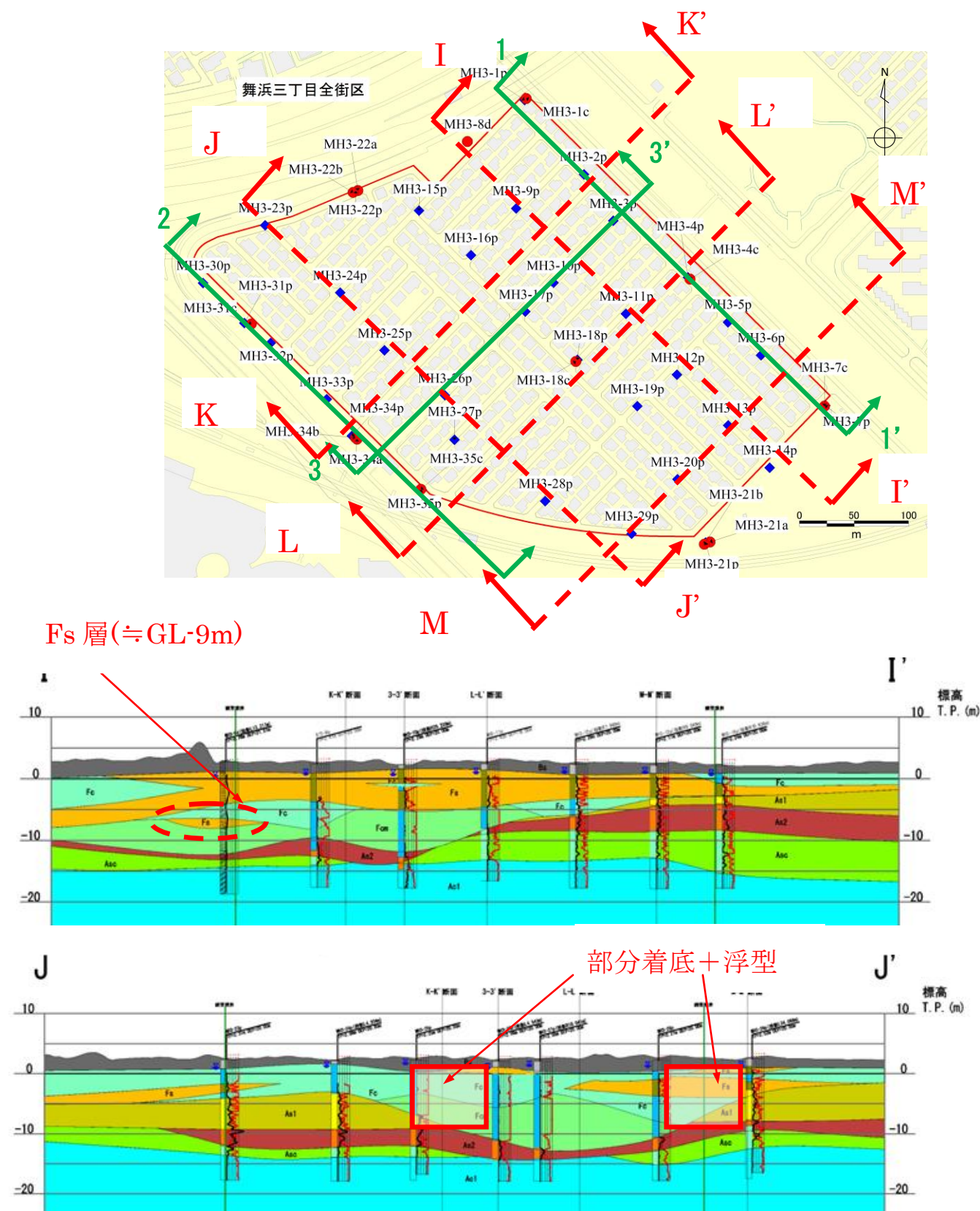
図-13.3 解析モデル作成断面と地下水位の設定
