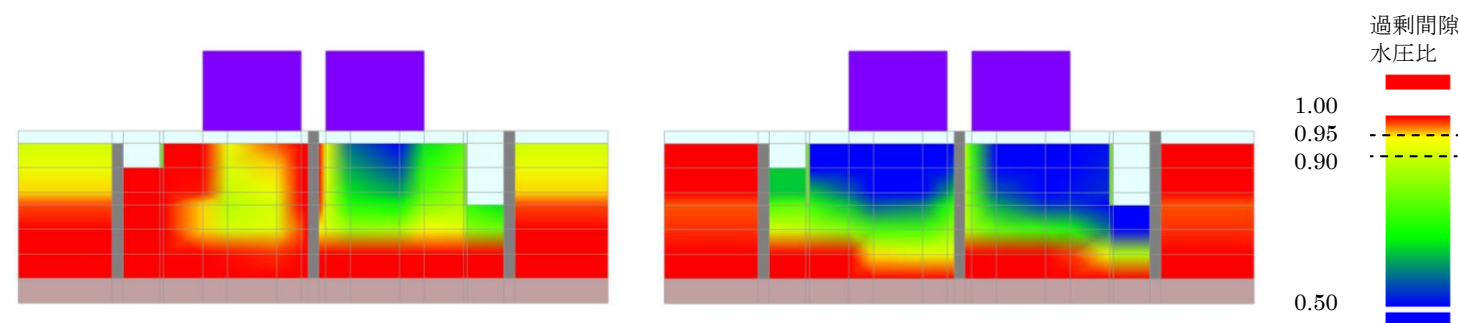
図-5.22 過剰間隙水圧比の最大値コンター(下水は加振直角方向) (左: Case-14、右: Case-15)
