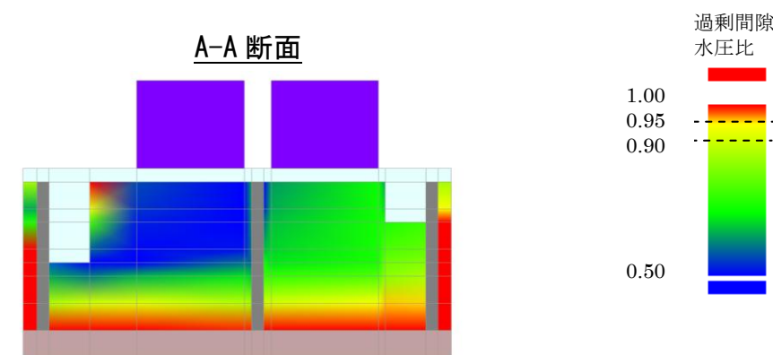
図-5.23 過剰間隙水圧比の最大値コンター (下水は加振平行方向、Case-16)
