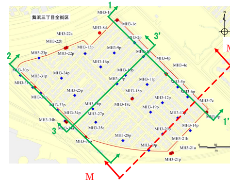
図-13.21 非液状化層厚 H1 の水平分布(M-M' 断面)
