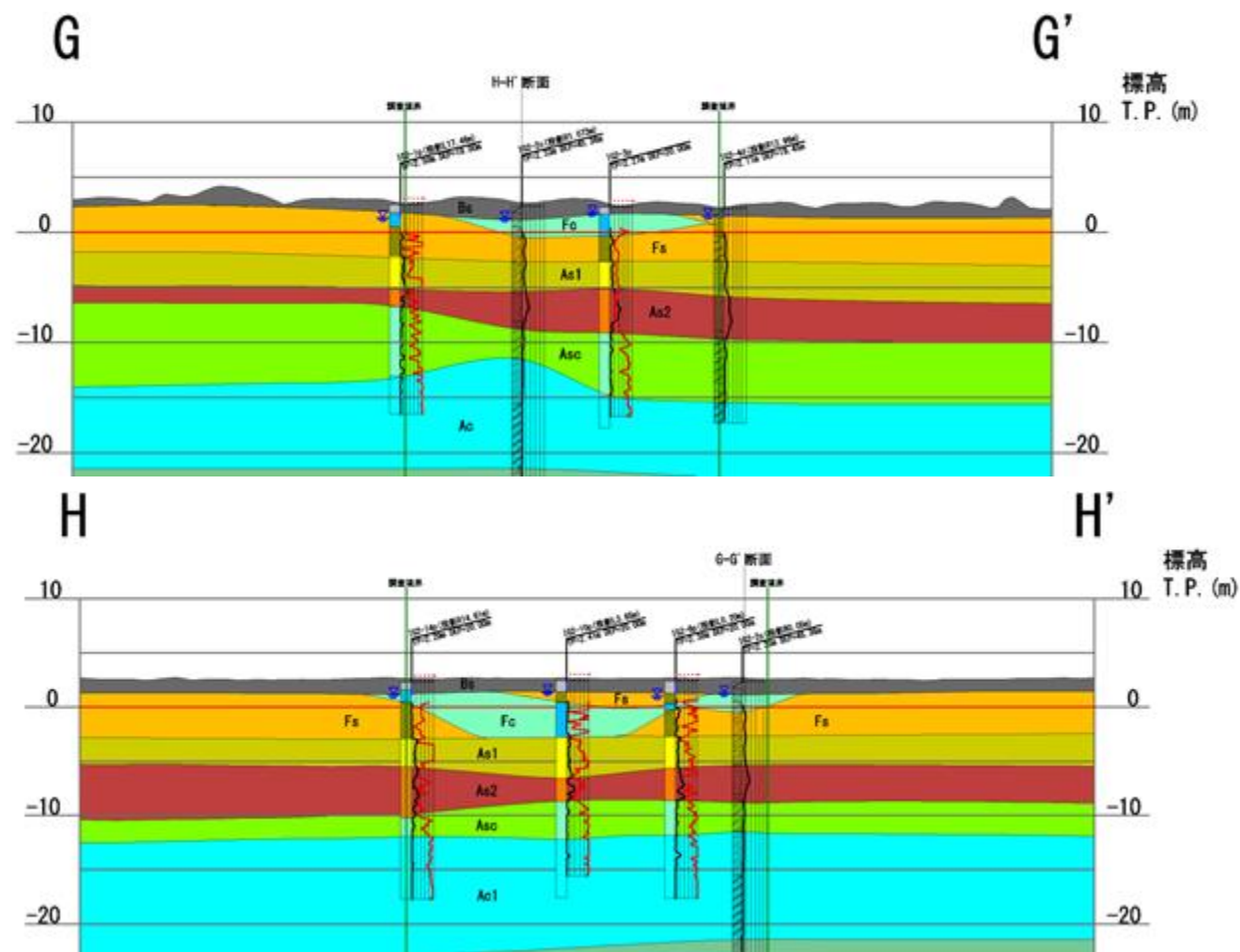
図-14.4 解析モデル作成断面
