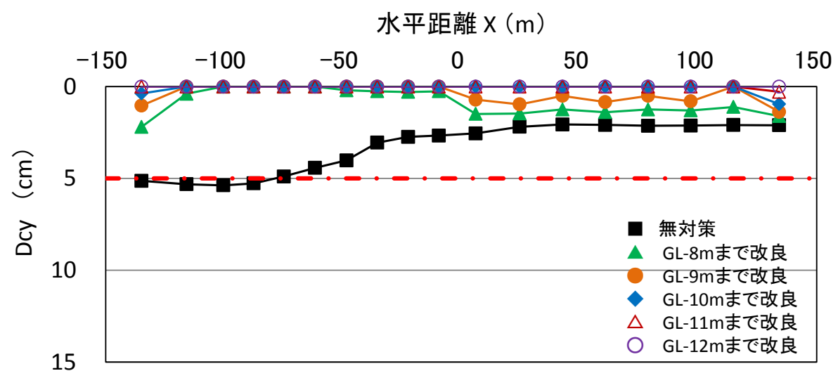
図-12.9 Dcyの水平分布 (F-F' 断面)
