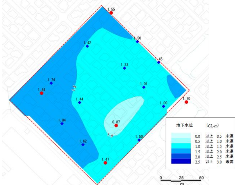
図-11.1 地下水位の計測結果
