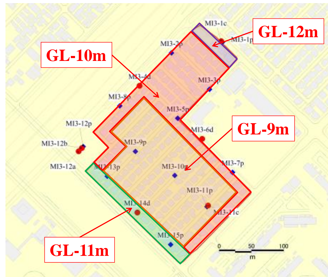
図-12.4 格子状地盤改良下端深度の平面分布図
