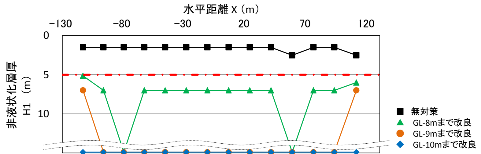
図-12.8 非液化化層厚 H1 の水平分布 (E-E' 断面)
