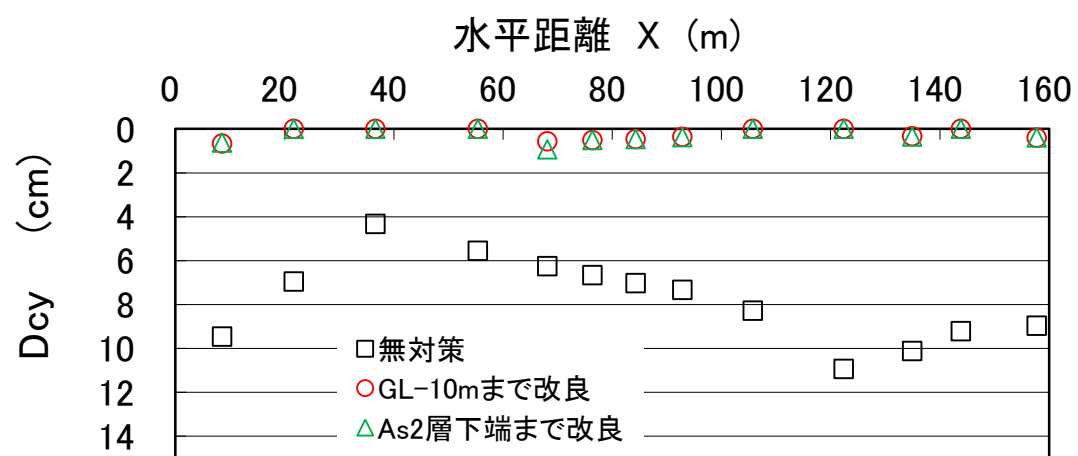
図-14.10 Dcyの水平分布(H-H'断面)
