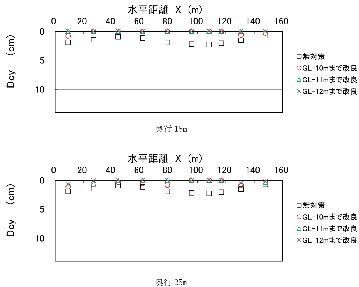
図-11.7 D_{cy} の水平分布 (A-A' 断面)
