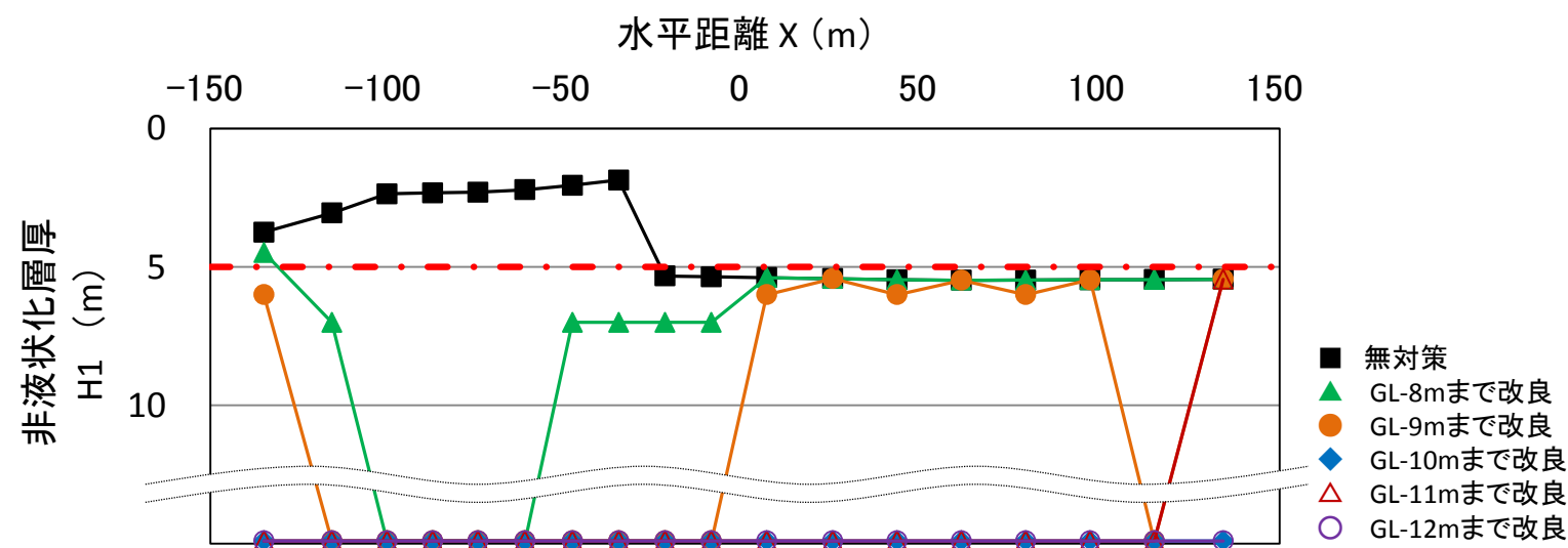
図-12.10 非液状化層厚 H1の水平分布 (F-F' 断面)
