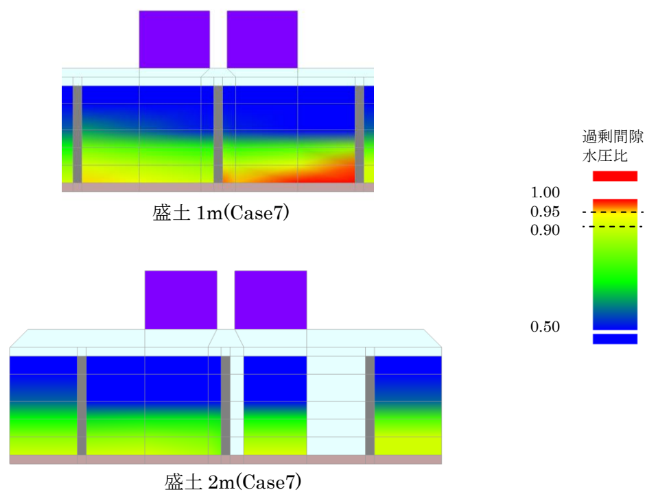
図-5.15 Case7の過剰間隙水圧比最大値コンター
