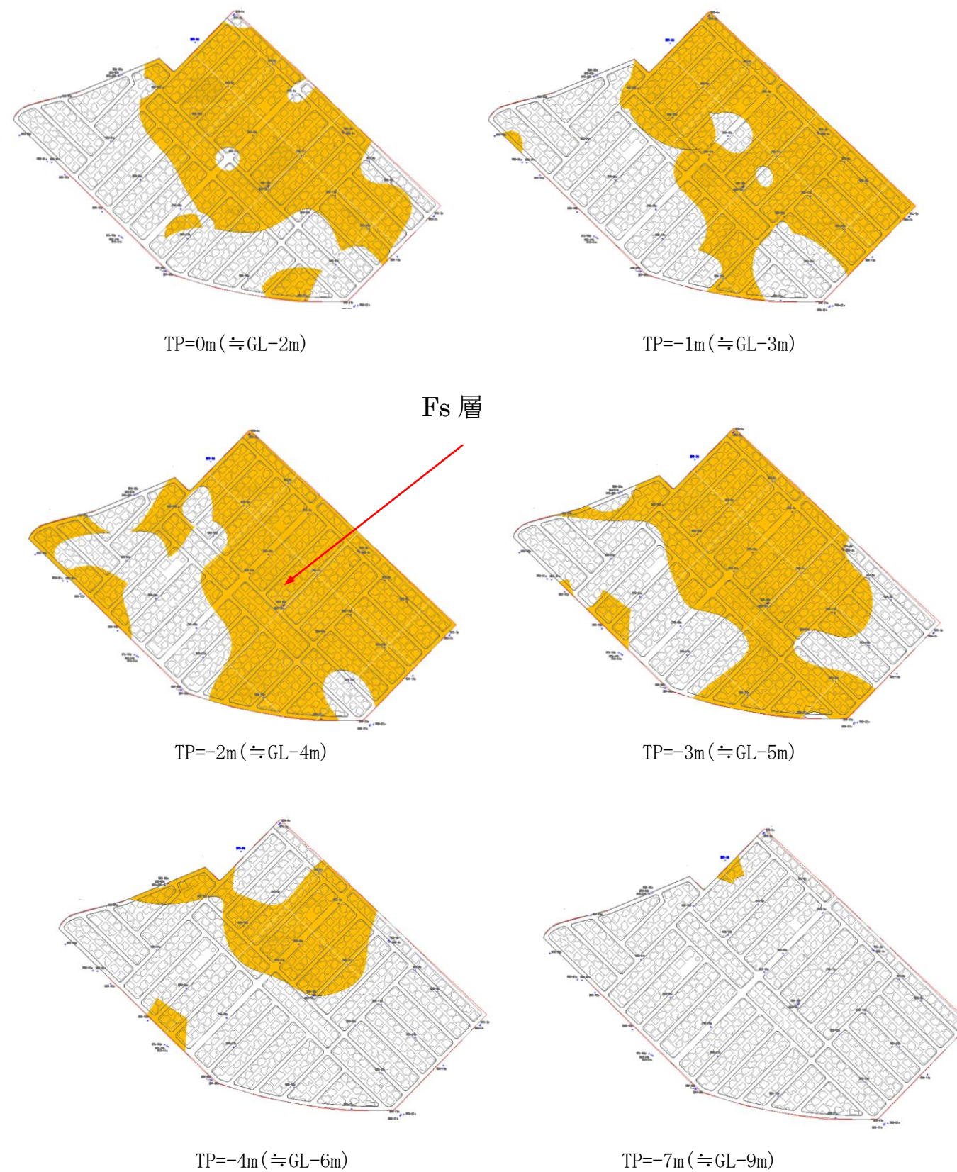
図-13.5 Fs層の平面分布図
