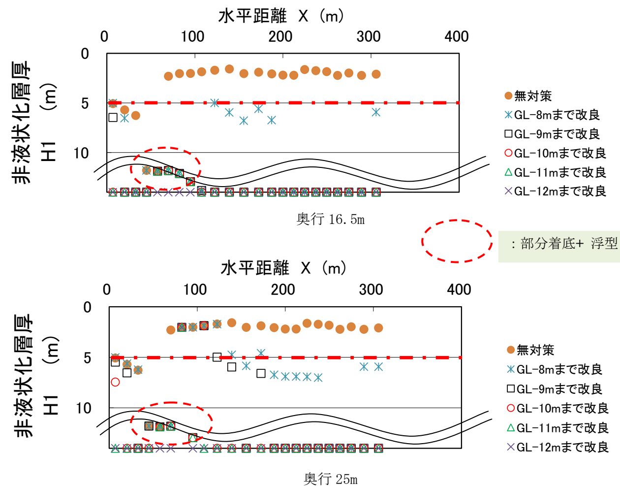
図-13.17 非液状化層厚 H1 の水平分布(K-K' 断面)
