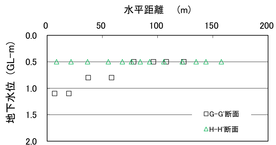
図-14.5 解析で設定した地下水位
