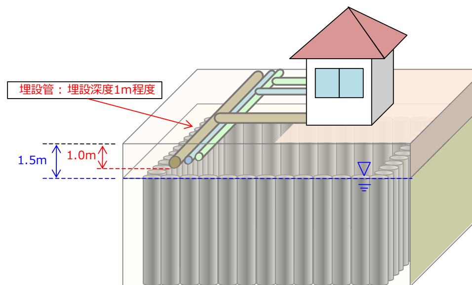
図-9.2 改良上端深度設定の概要図
