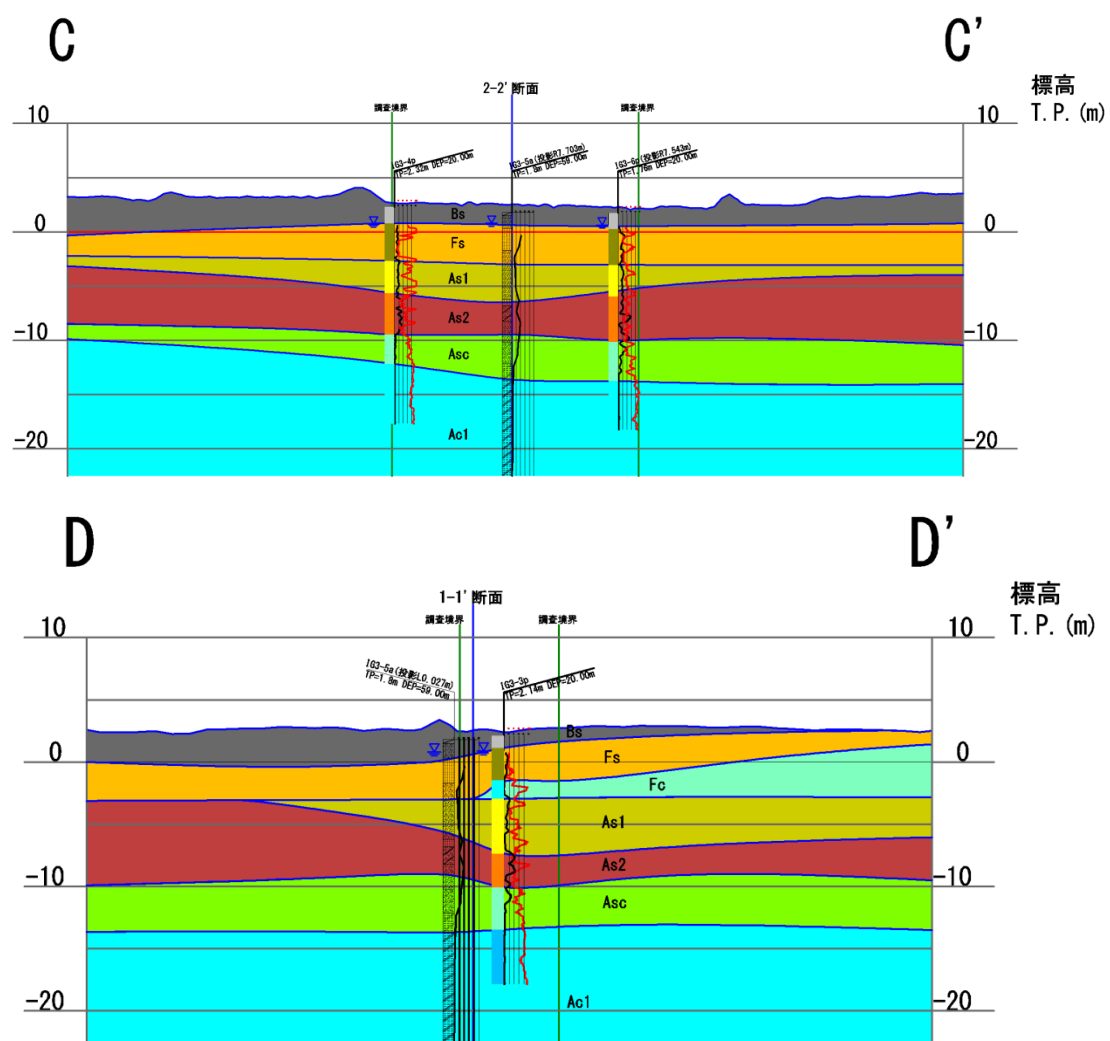
図-10.4 解析モデル作成断面
