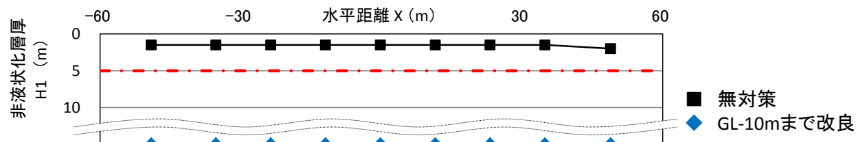
図-10.10 非液状化層厚 H1の水平分布 (C-C' 断面)
