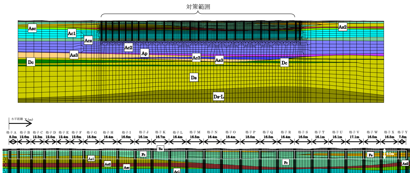
図-13.8 J-J' 断面の解析モデル(上：全体モデル、下：対策範囲を拡大)
