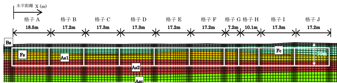
図-11.7 D_{cy} の水平分布 (A-A' 断面)
