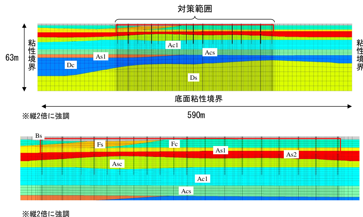
図-12.6 F-F' 断面の擬似 3 次元解析モデル (上: 全体、下: 対策範囲拡大)
