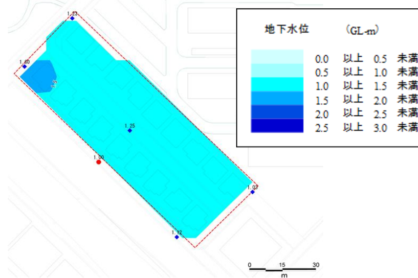
図-10.2 地下水水位の計測結果
