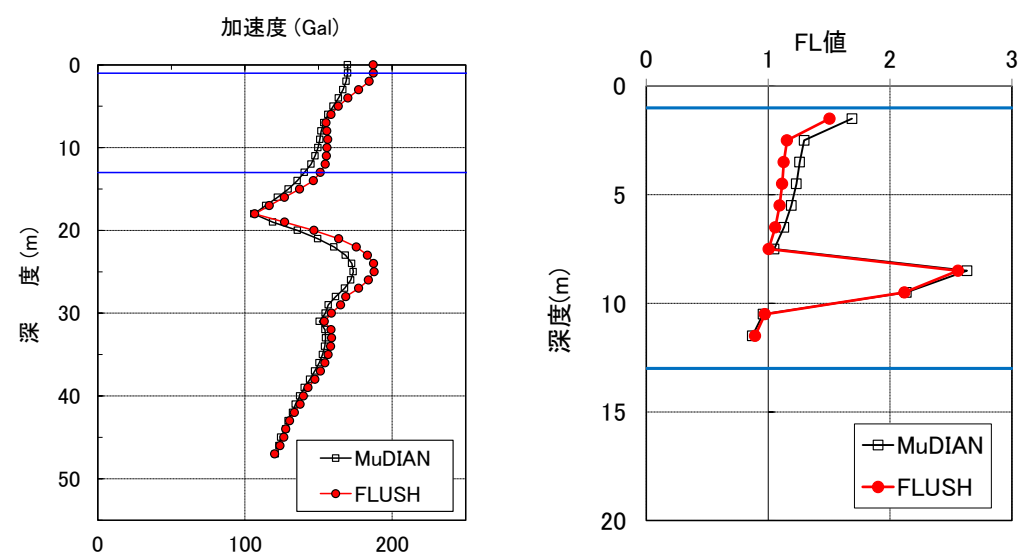
図-4.9 16m×16mの格子内地盤中央での加速度とFL値深度分布(解析コードの比較)
