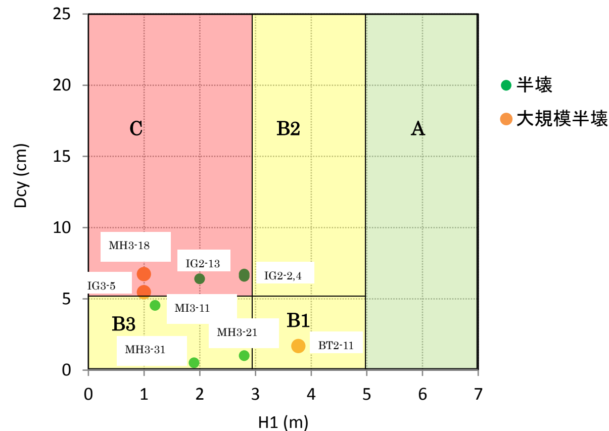
図-8.7 1次元等価線形解析で求めた非液状化層厚H1とDcyの関係 (液状化抵抗は各層の平均Naから算出)
