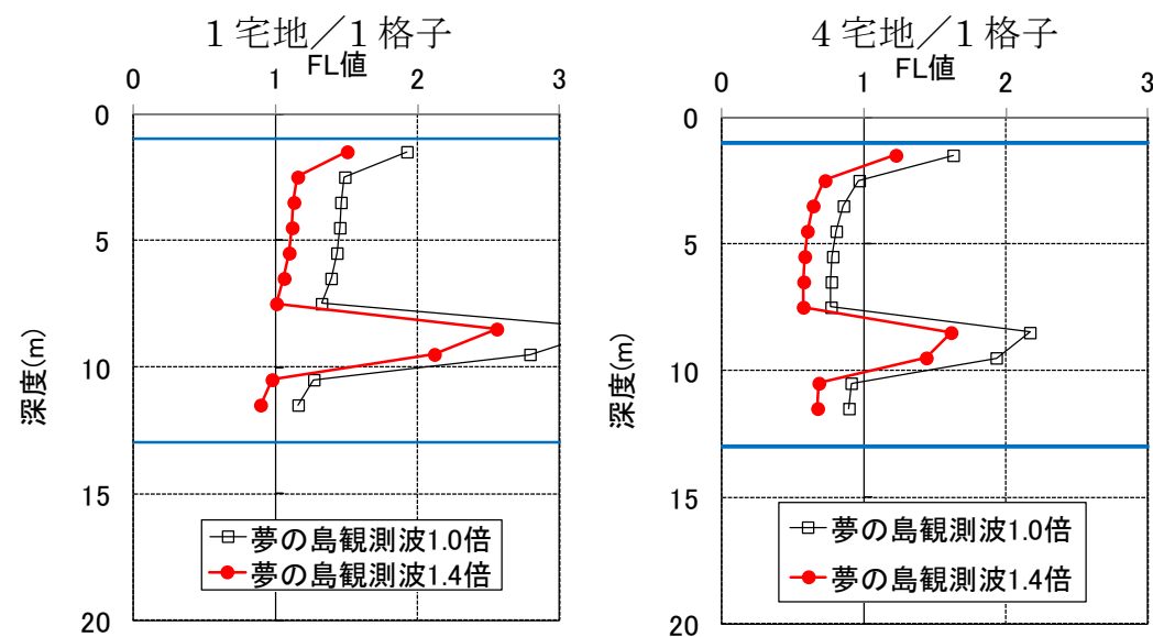
図-4.6 対策後のFL値の深度分布 (「液状化対策実現可能性検討委員会(平成24年)」)
