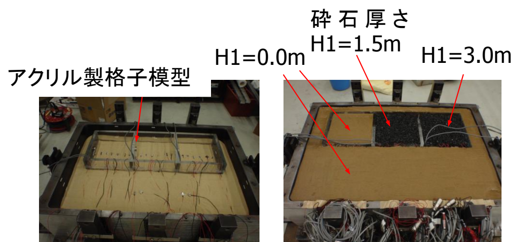
図-5.11 模型地盤の作成状況
