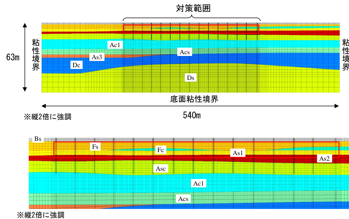
図-12.5 E-E' 断面の擬似 3 次元解析モデル (上: 全体、下: 対策範囲拡大)
