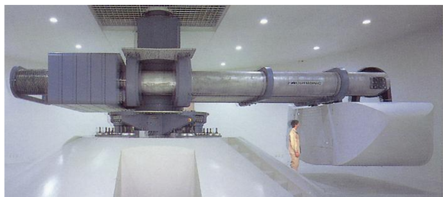
図-5.1 遠心実験装置全景(竹中技術研究所)
