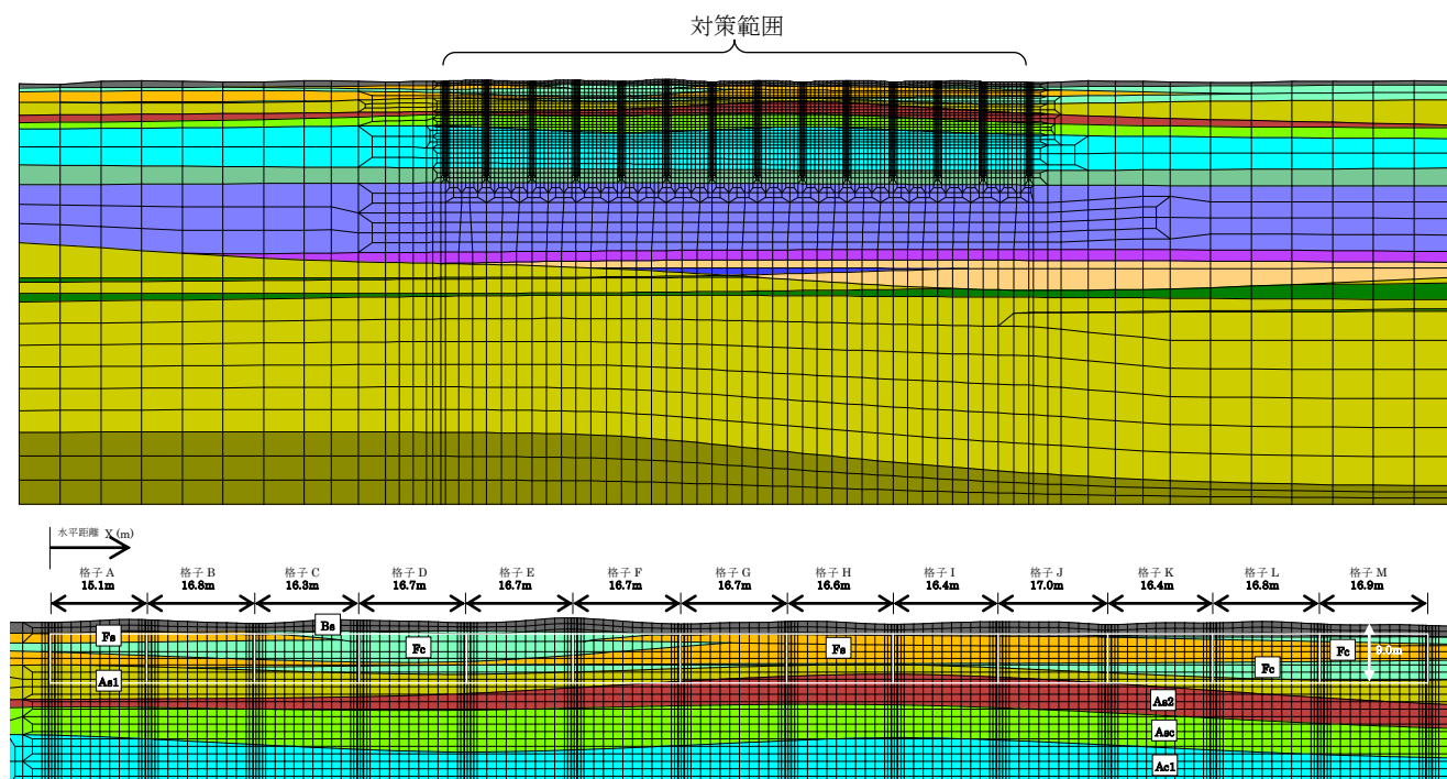
図-13.11 M-M' 断面の解析モデル(上：全体モデル、下：対策範囲を拡大)
