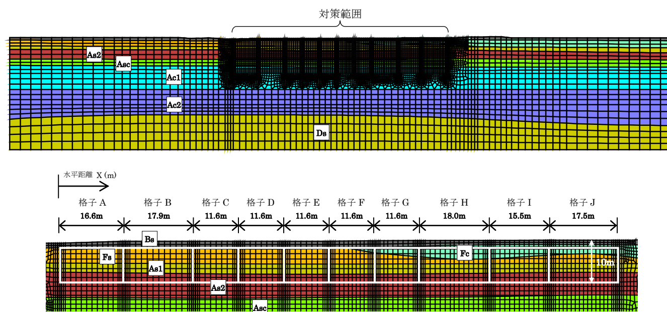
図-11.6 B-B' 断面の解析モデル(上：全体モデル、下：対策範囲を拡大)
