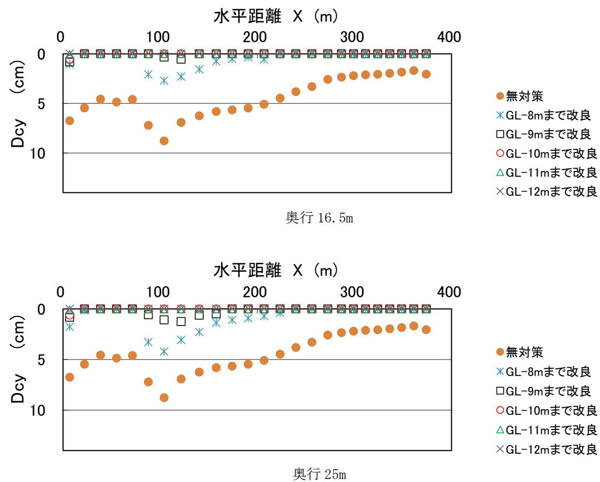
図-13.12 D_{cy} の水平分布 (I-I' 断面)
