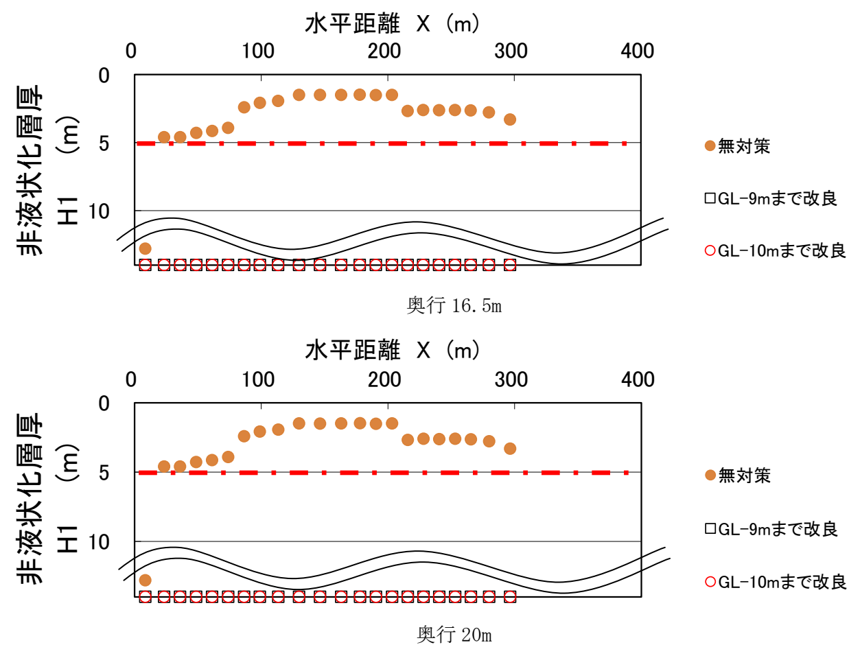
図-13.19 非液状化層厚H1の水平分布(L-L'断面)
