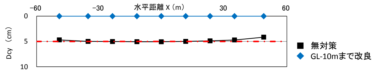
図-10.9 Dcyの水平分布 (C-C' 断面)
