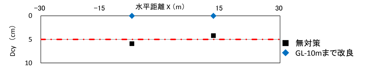
図-10.11 Dcyの水平分布 (D-D' 断面、奥行17m)
