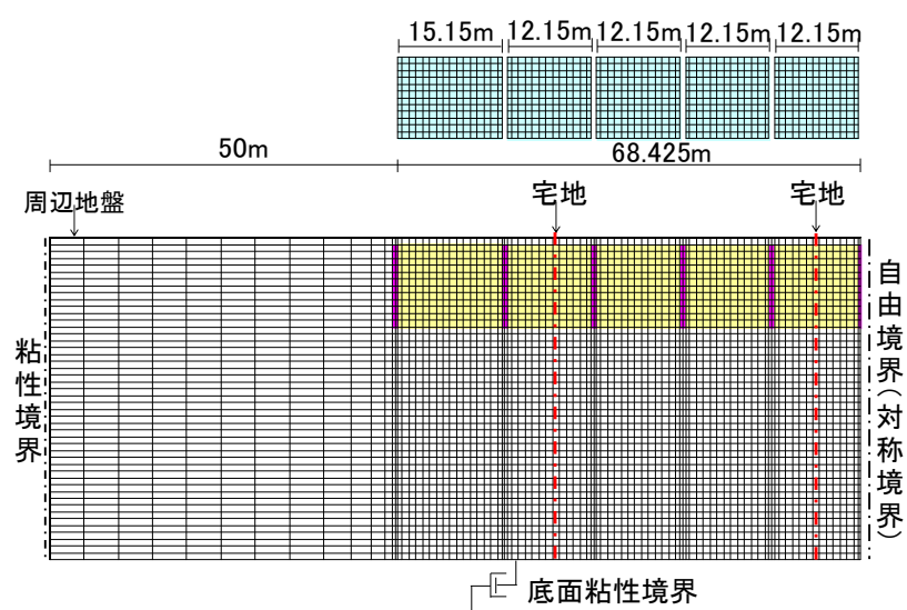
図-4.4 モデル地盤の解析モデル(1つの格子で1つの宅地と道路を対策) (「液状化対策実現可能性検討委員会(平成24年)」)
