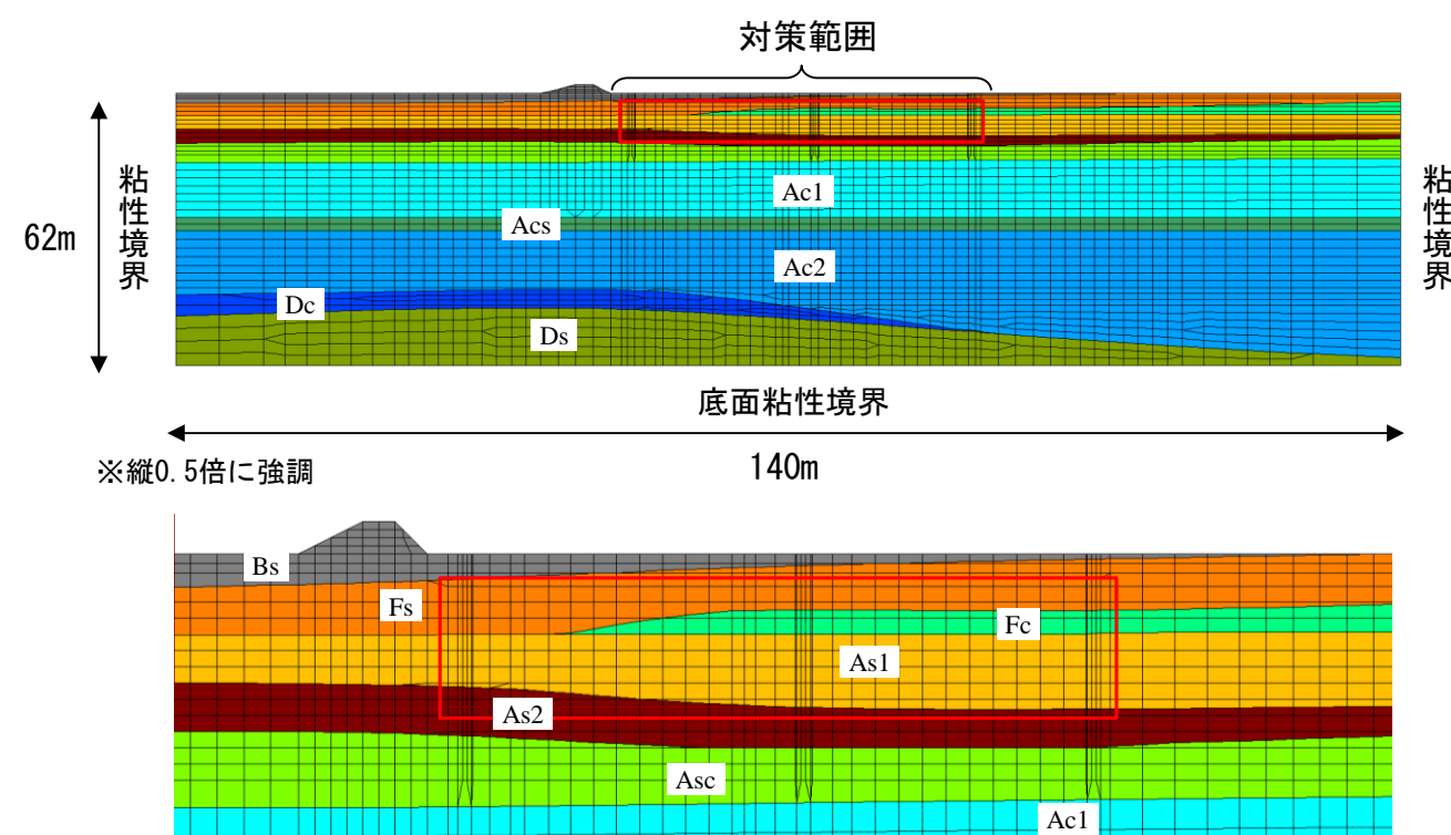
図-10.8 D-D'断面の擬似3次元解析モデル(上:全体、下:対策範囲拡大)
