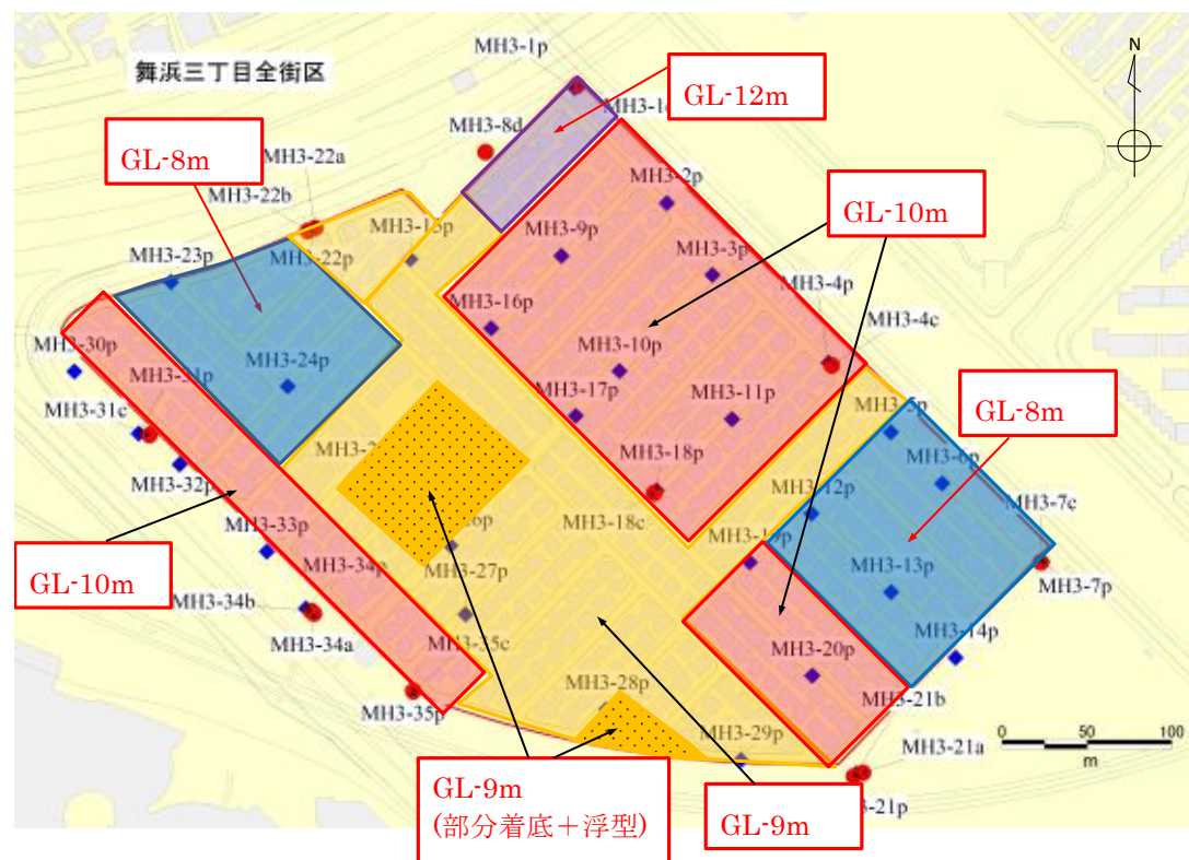
図-13.4 格子壁下端深度の平面分布図
