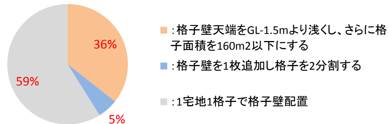
図-14.3 対策対象地震動に対してFL>1.0を満足できる条件
