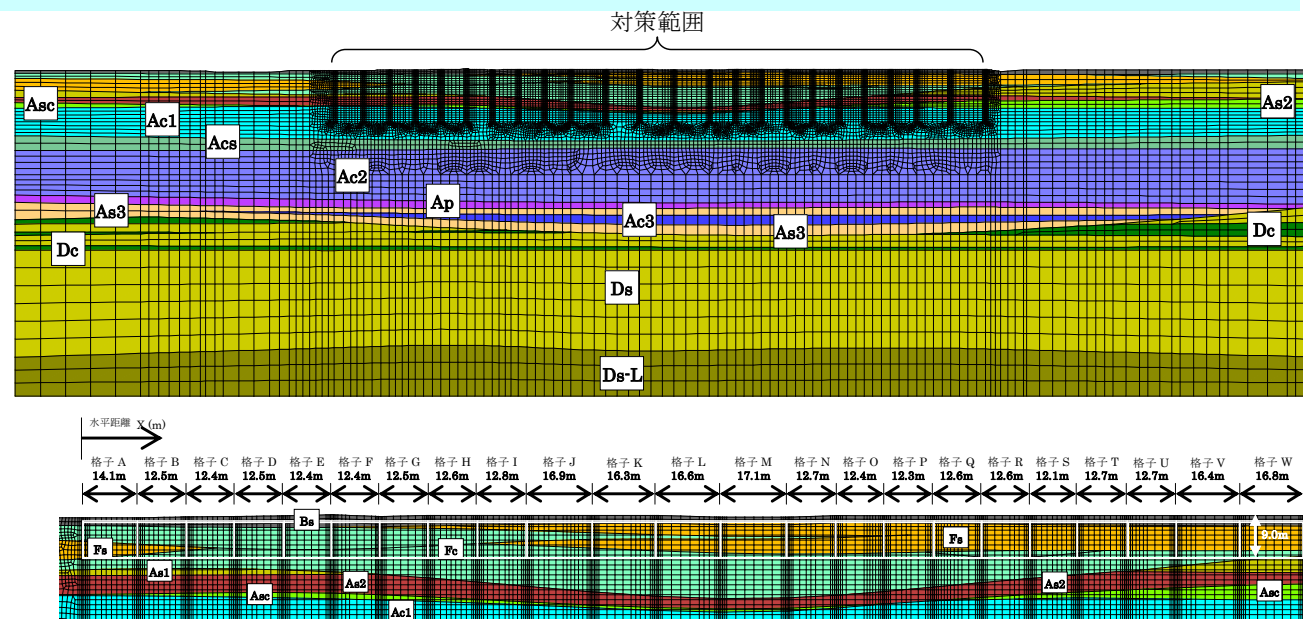
図-13.9 K-K' 断面の解析モデル(上：全体モデル、下：対策範囲を拡大)
