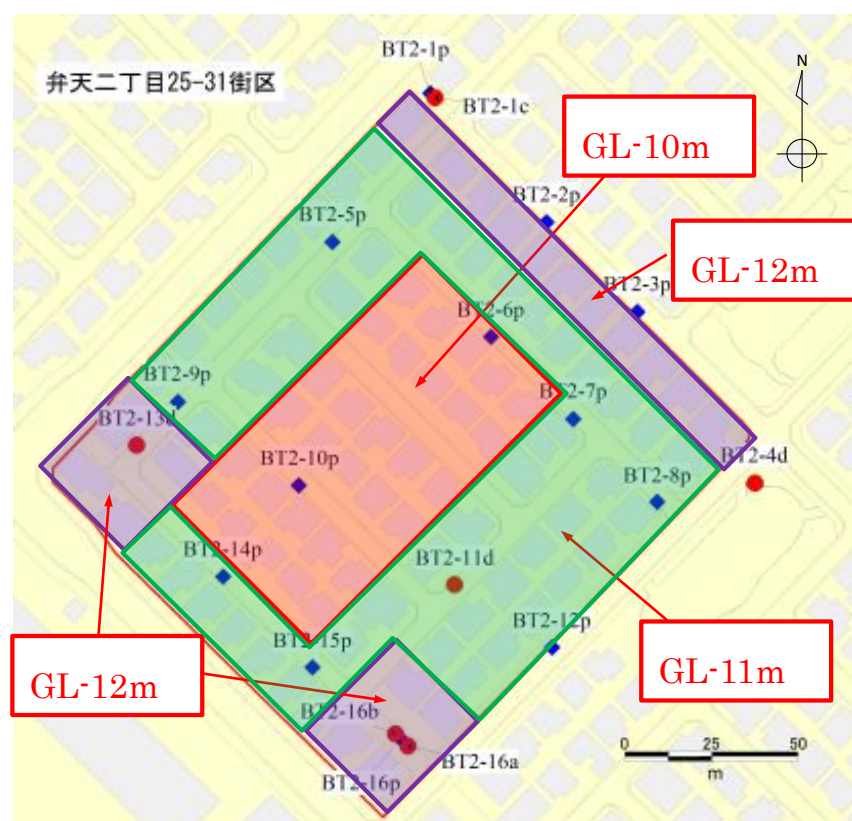
図-11.4 FL 値 > 1.0 を満足する改良仕様の平面分布図(対策対象地震動、調査宅地を対象)
