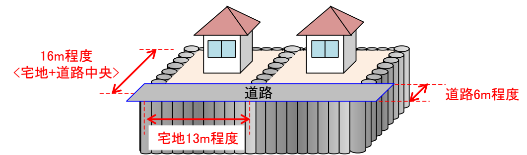
図-6.2 格子状地盤改良工法での基本配置
