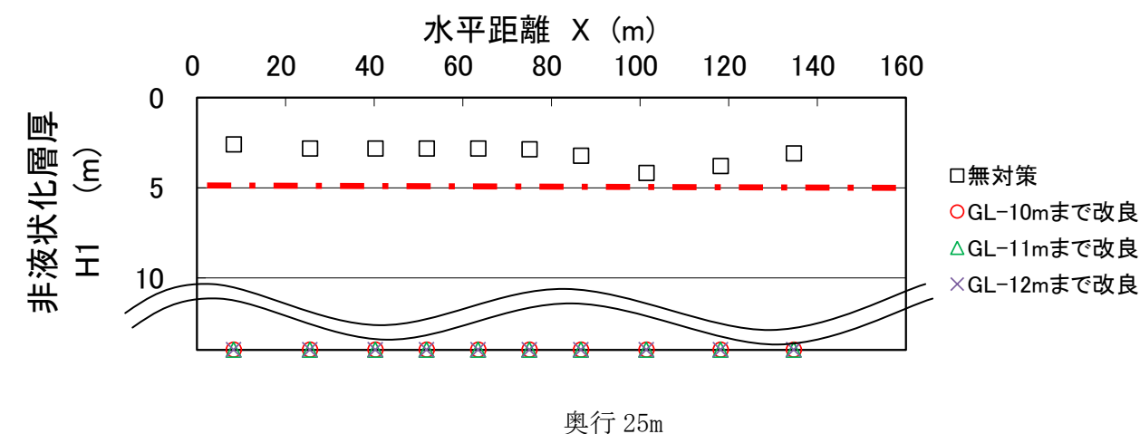
図-11.10 非液状化層厚 H1 の水平分布 (B-B' 断面)
