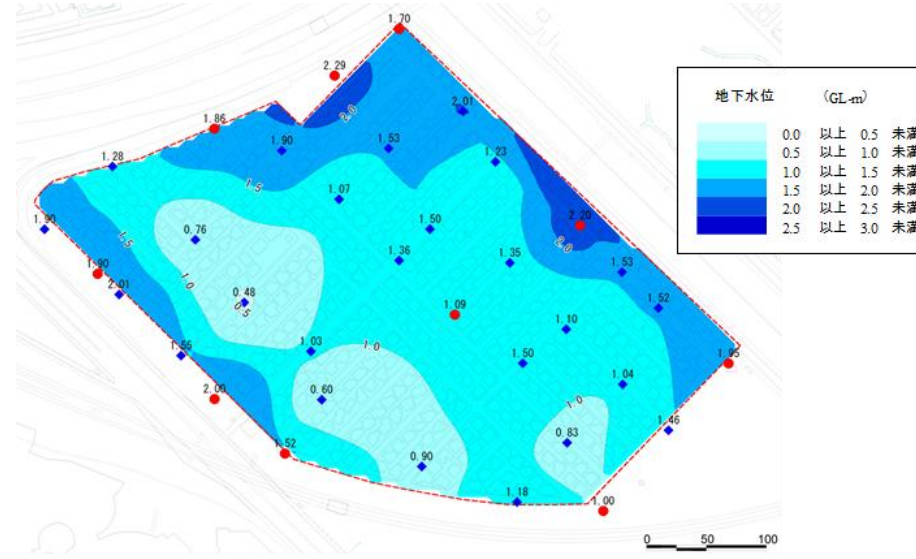
図-13.1 地下水位の計測結果
