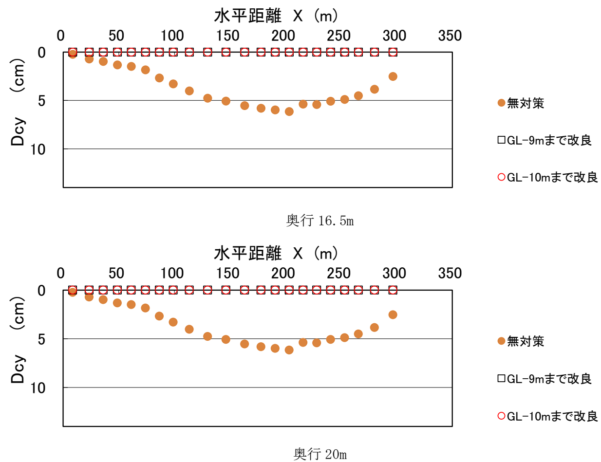
図-13.18 Dcyの水平分布(L-L'断面)
