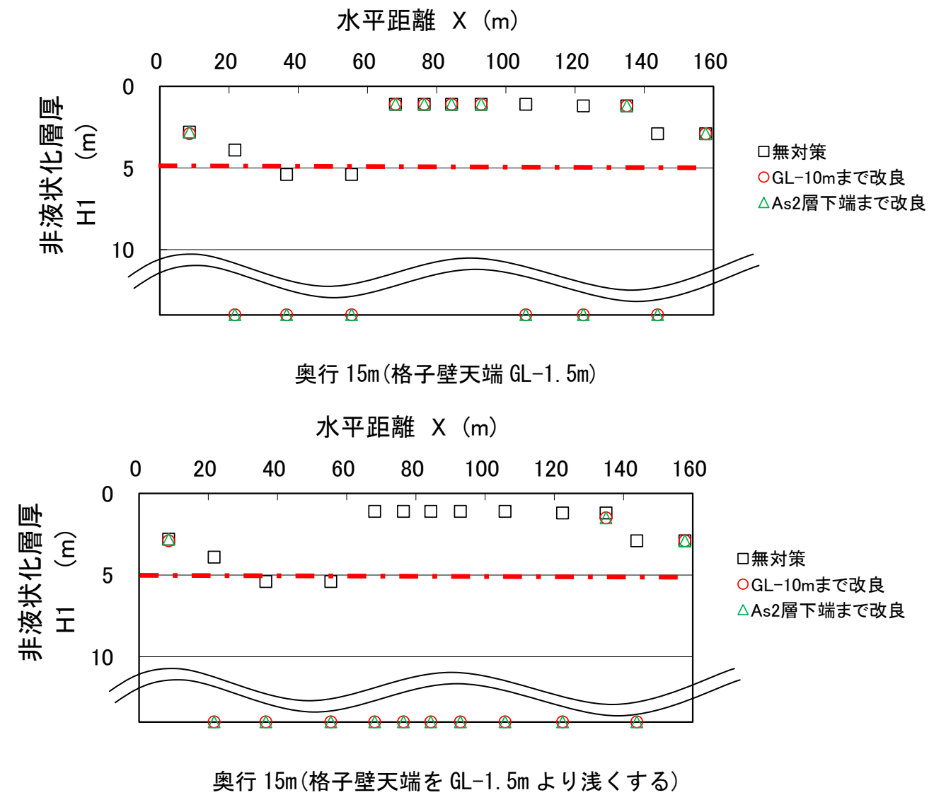
図-14.12 非液状化層厚 H1 の水平分布(H-H' 断面、奥行 15m)
