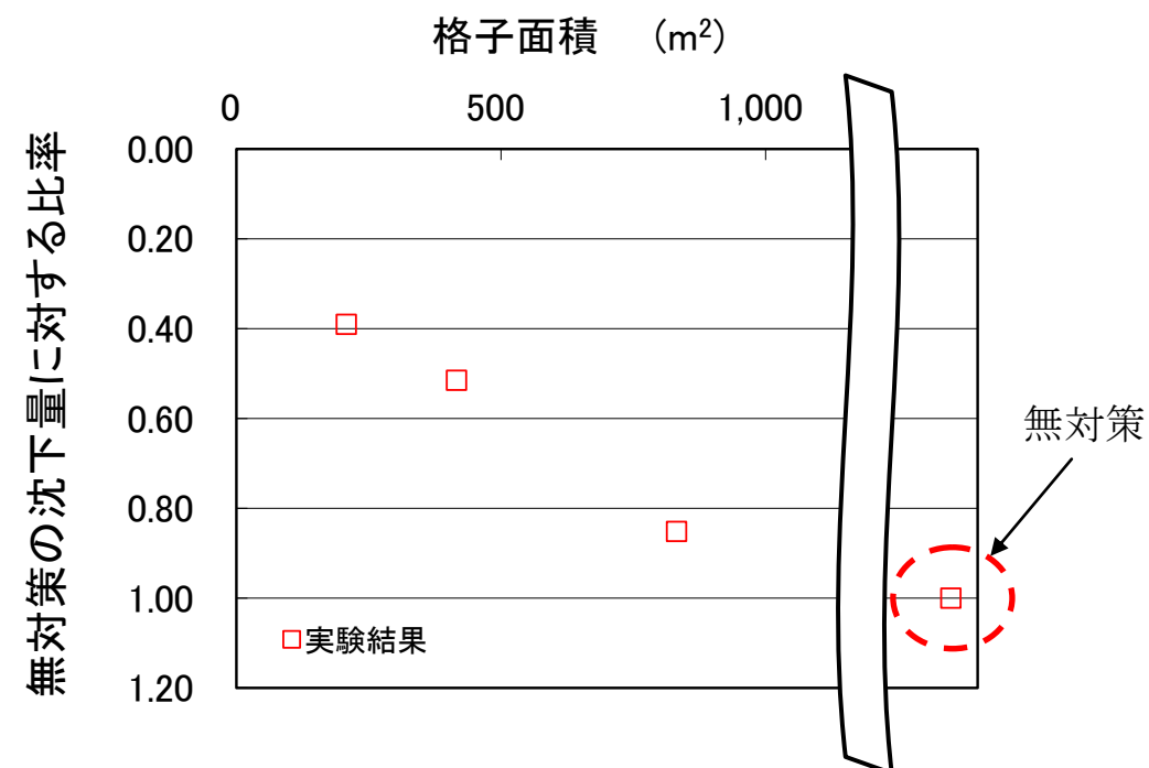
図-5.6 格子面積と沈下量の関係
