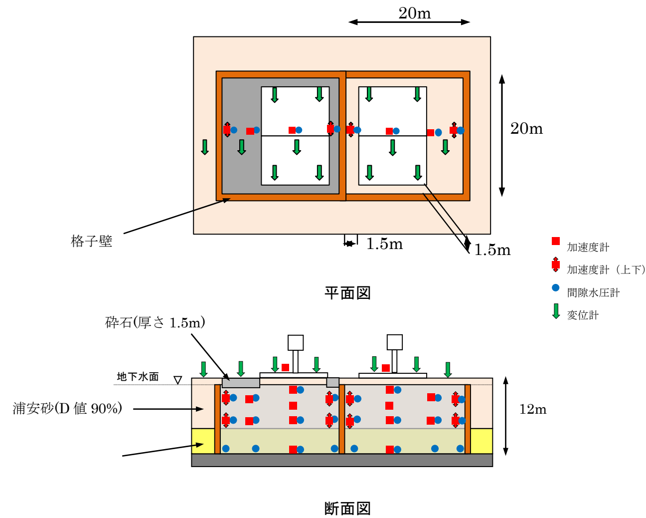
図-5.17 格子間隔20m×20mの模型地盤(左:住宅周囲碎石厚1.5m、右:碎石なし)
