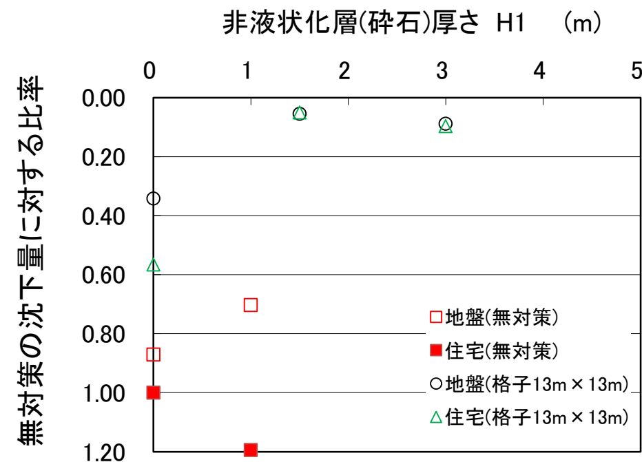
図-5.12 非液状化層厚と住宅・地表面沈下量の関係
