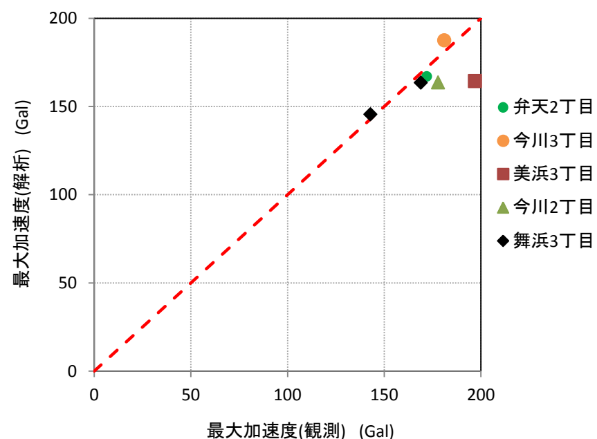
図-8.5 地表面加速度の1次元等価線形解析結果と観測結果の比較 (弁天2丁目は夢の島1.3倍振幅、他4地区は夢の島1.1倍振幅での設定振幅を使用)
