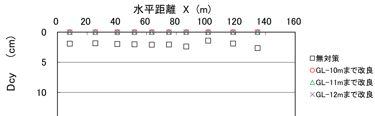
図-11.9 Dcy の水平分布 (B-B' 断面)
