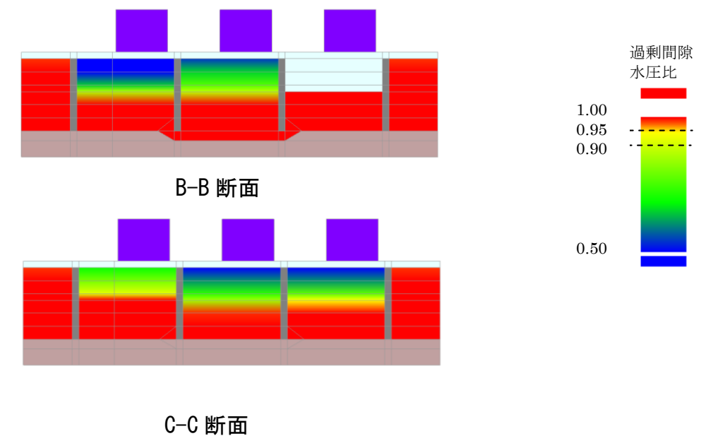
図-5.27 Case-17の過剰間隙水圧比の最大値コンター
