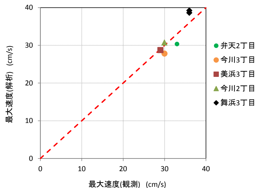
図-8.6 地表面速度の1次元等価線形解析結果と観測結果の比較 (弁天2丁目は夢の島1.3倍振幅、他4地区は夢の島1.1倍振幅での設定振幅を使用)
