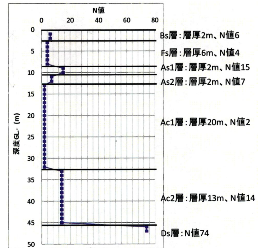
図-4.2 モデル地盤(地下水位 GL-1m) (「液状化対策実現可能性検討委員会(平成24年)」)
