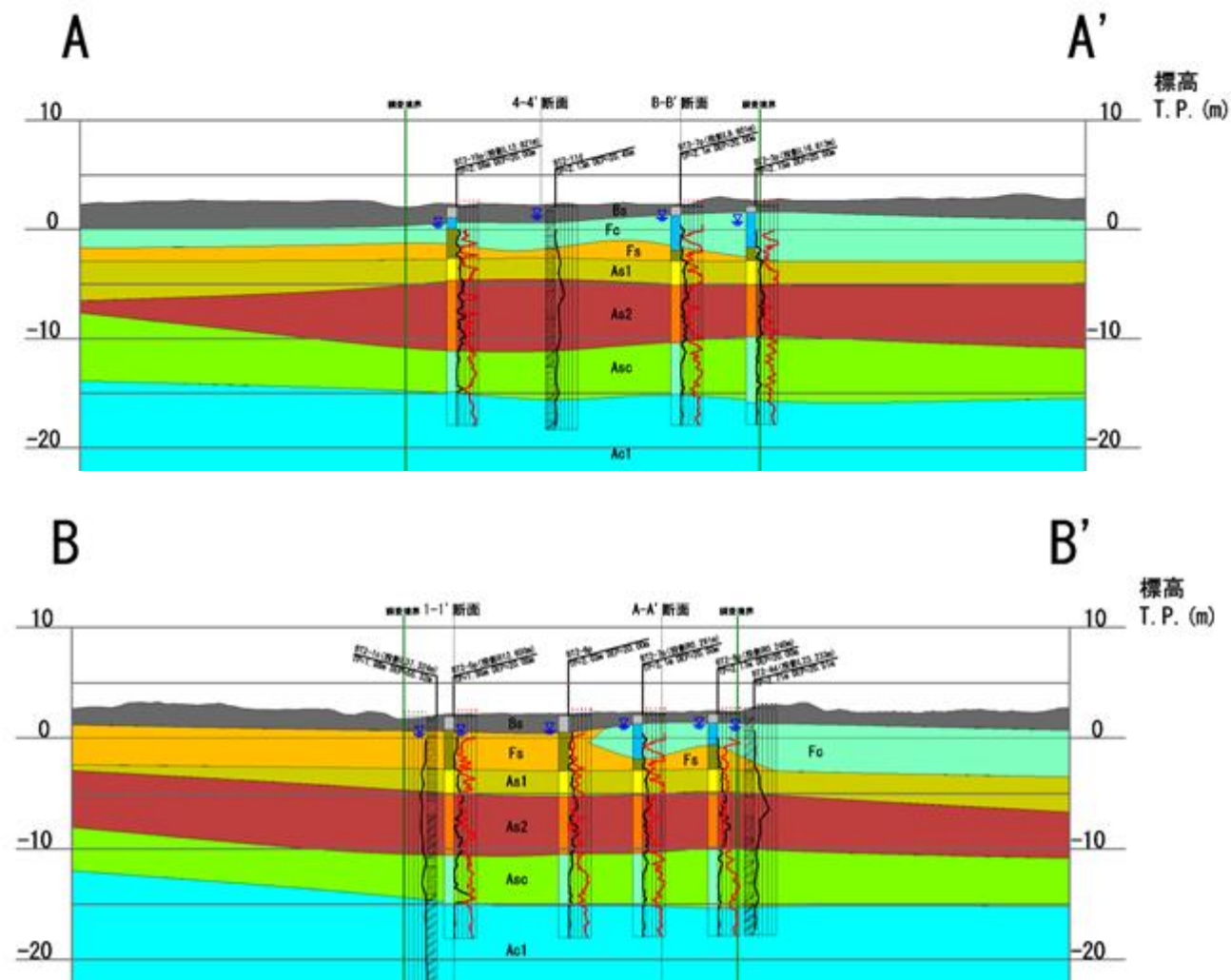
図-11.3 解析モデル作成断面
