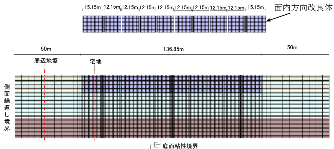
図-4.7 MuDIANの等価線形解析モデル(擬似3次元)
