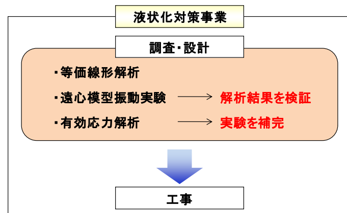
図-4.1 液状化対策事業での性能照査の考え方
