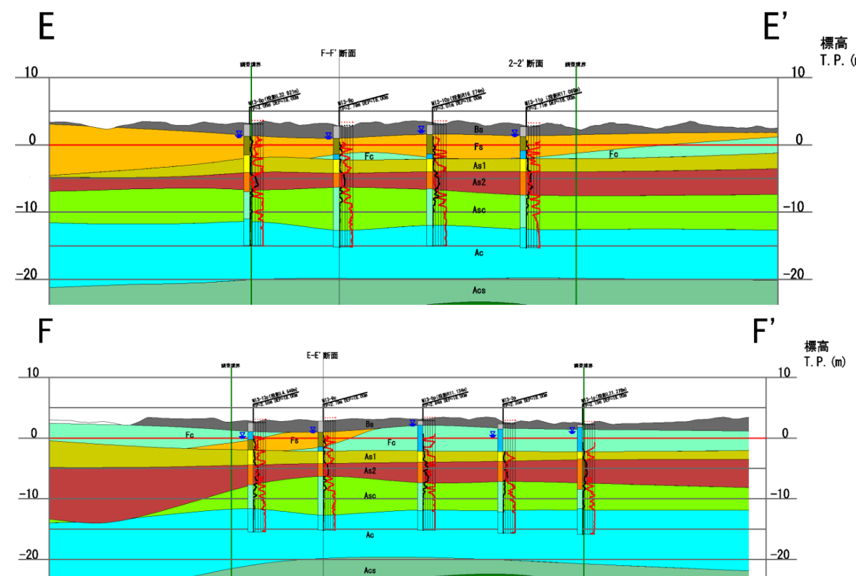
図-12.2 解析モデル作成断面
