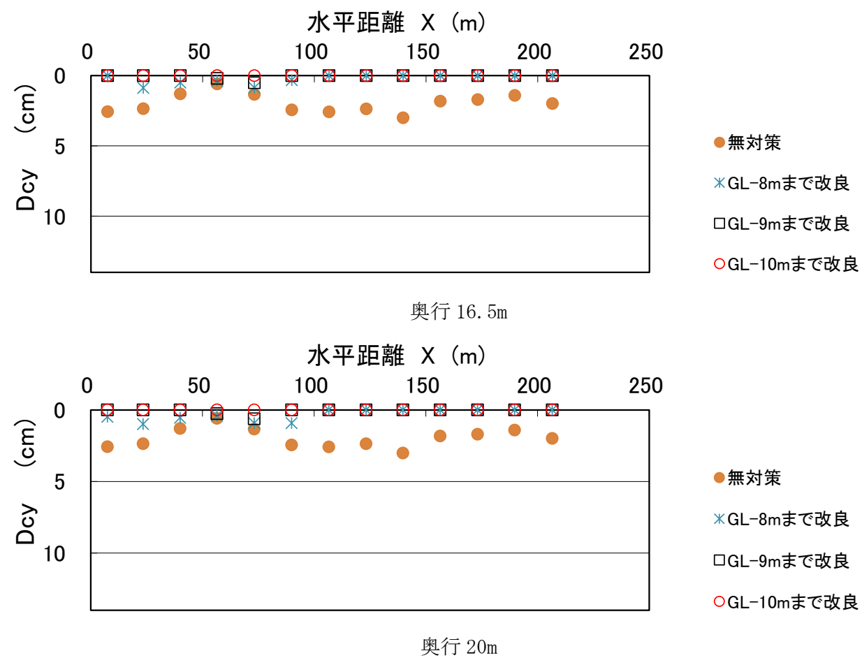
図-13.20 Dcy の水平分布(M-M' 断面)
