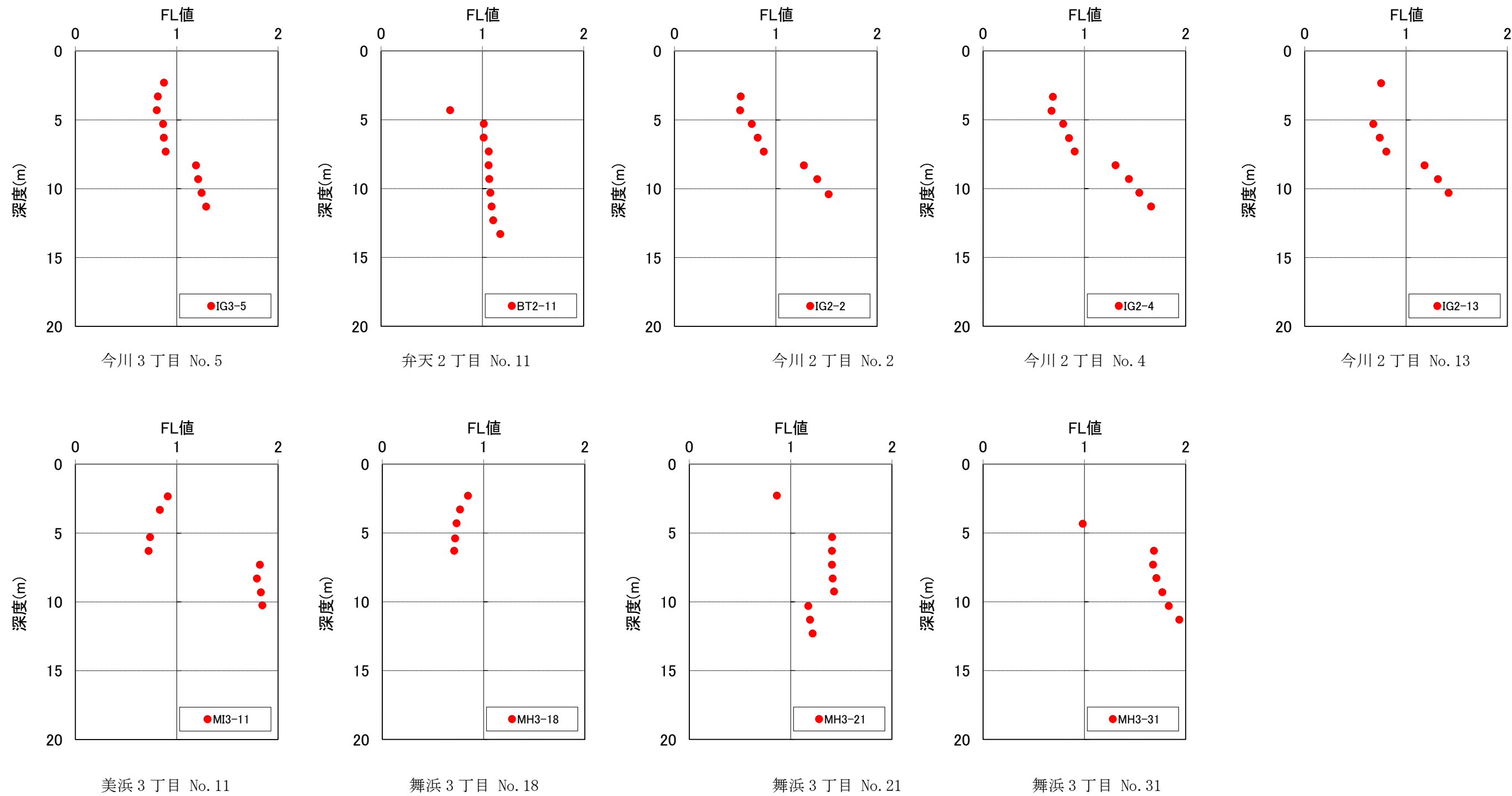
図-8.8 1次元等価線形解析結果から求めた各地区のFL値深度分布
