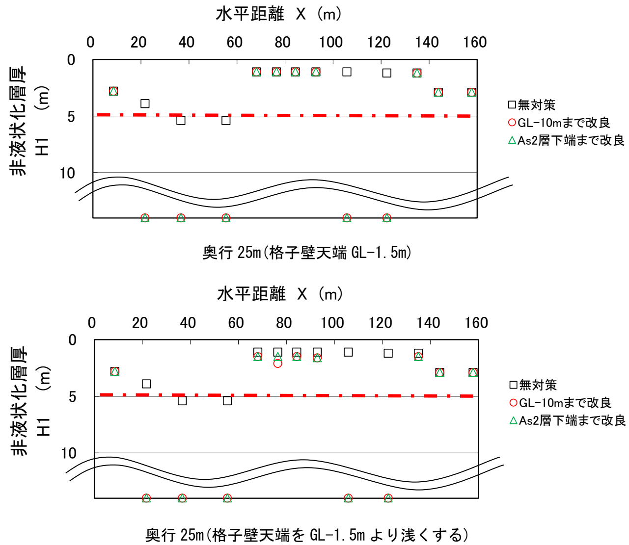
図-14.11 非液状化層厚 H1 の水平分布(H-H' 断面、奥行 25m)
