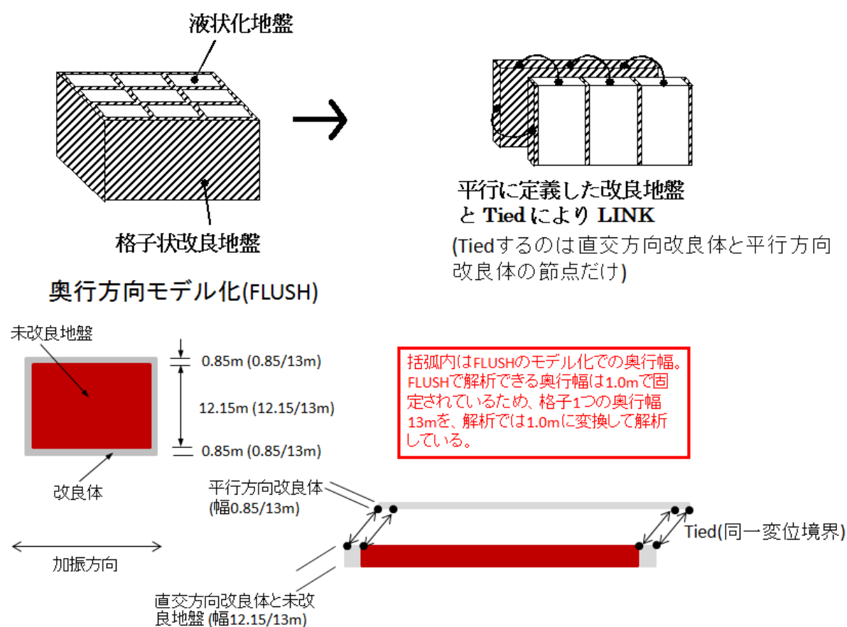
図-4.3 格子状地盤改良の擬似3次元モデルによるモデル化
