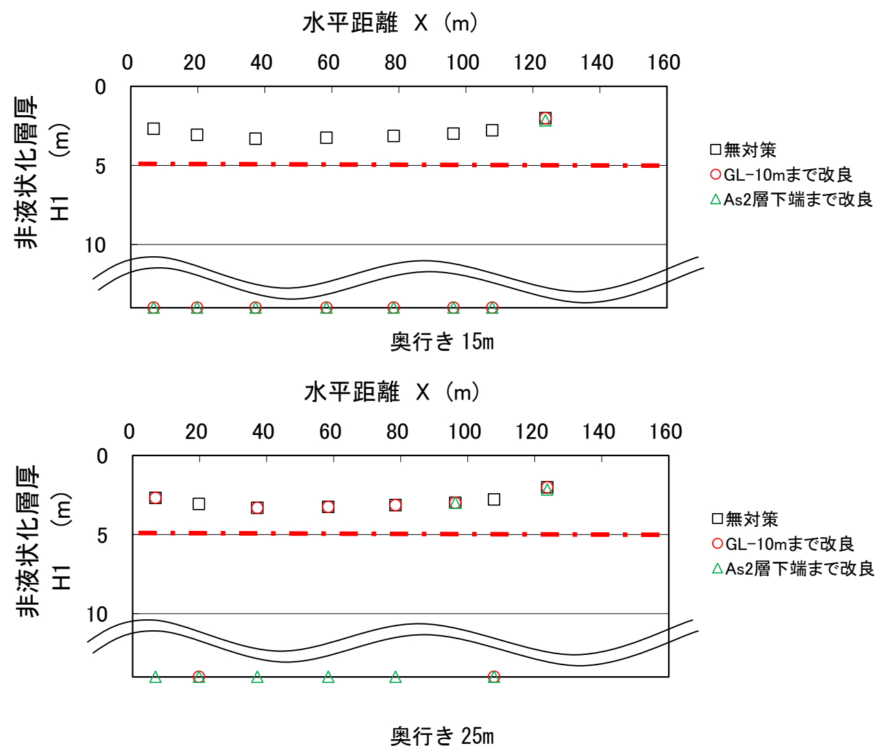
図-14.9 非液状化層厚 H1の水平分布(G-G'断面)
