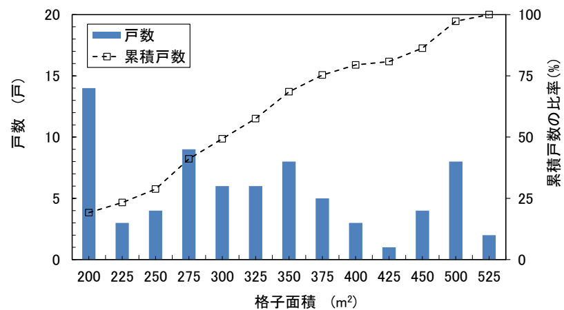
図-14.2 格子面積と累積戸数の関係
