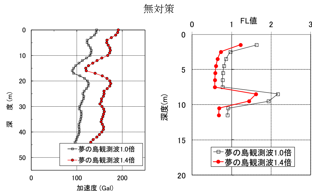
図-4.5 無対策での加速度とFL値の深度分布 (「液状化対策実現可能性検討委員会(平成24年)」)
