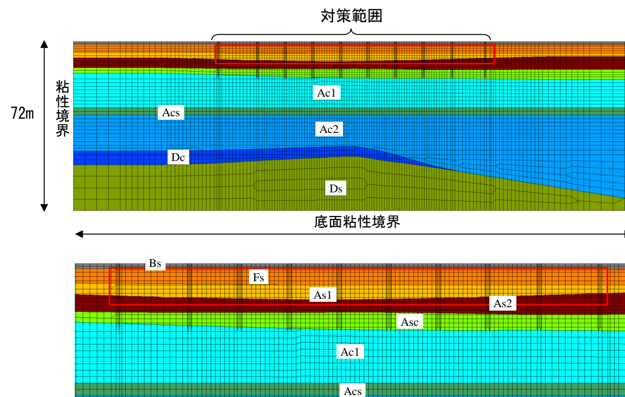
図-10.7 C-C'断面の擬似3次元解析モデル(上:全体、下:対策範囲拡大)
