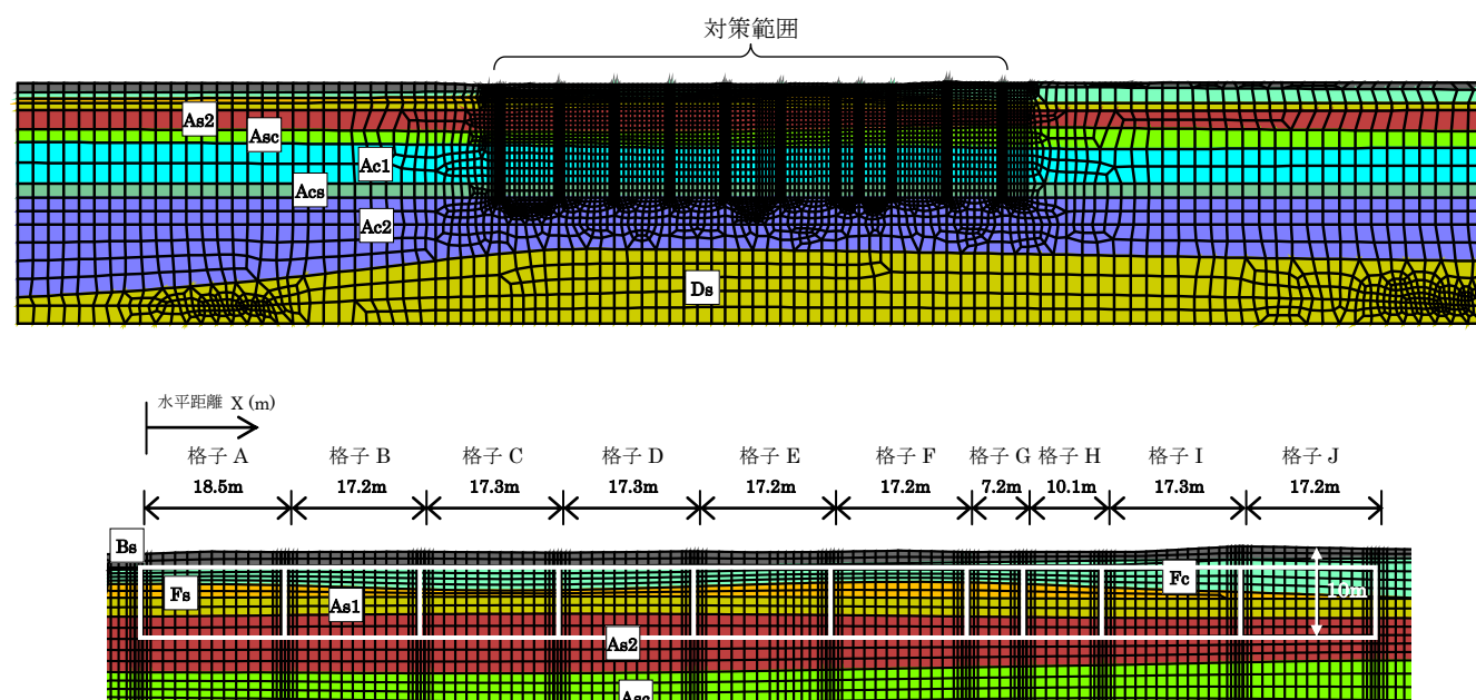
図-11.5 A-A' 断面の解析モデル(上：全体モデル、下：対策範囲を拡大)
