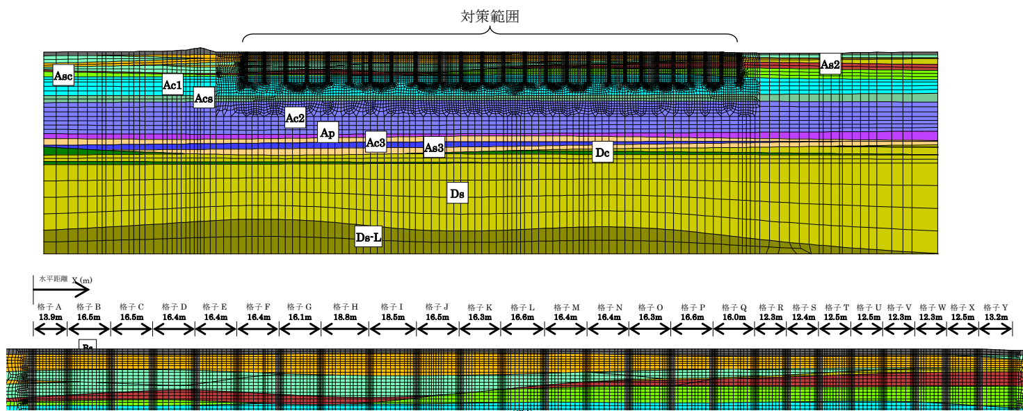
図-13.7 I-I' 断面の解析モデル(上：全体モデル、下：対策範囲を拡大)
