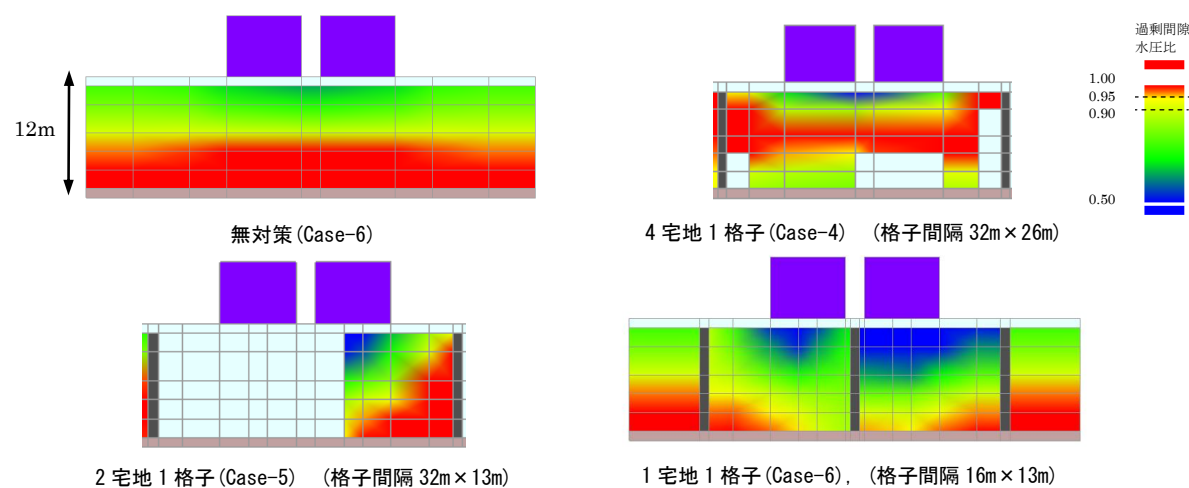
図-5.7 過剰間隙水圧比の最大値コンター図
