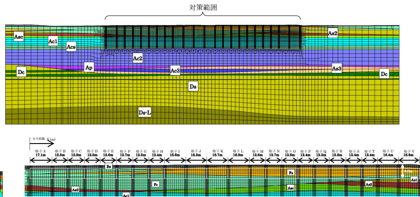
図-13.10 L-L' 断面の解析モデル(上：全体モデル、下：対策範囲を拡大)
