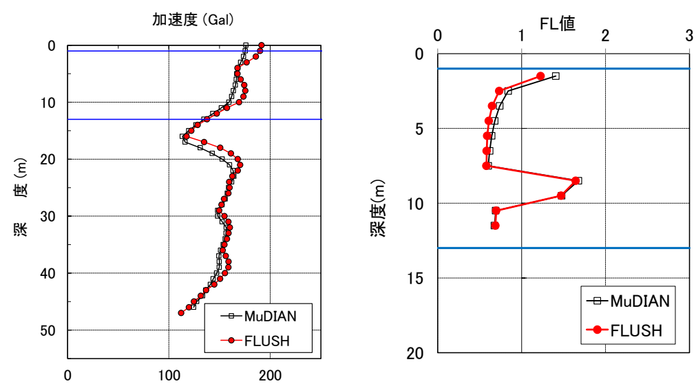
図-4.8 周辺地盤での加速度とFL値深度分布(解析コードの比較)
