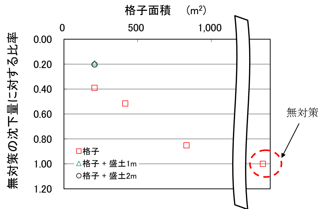
図-5.16 格子状地盤改良単独と盛土併用の住宅沈下量比較
