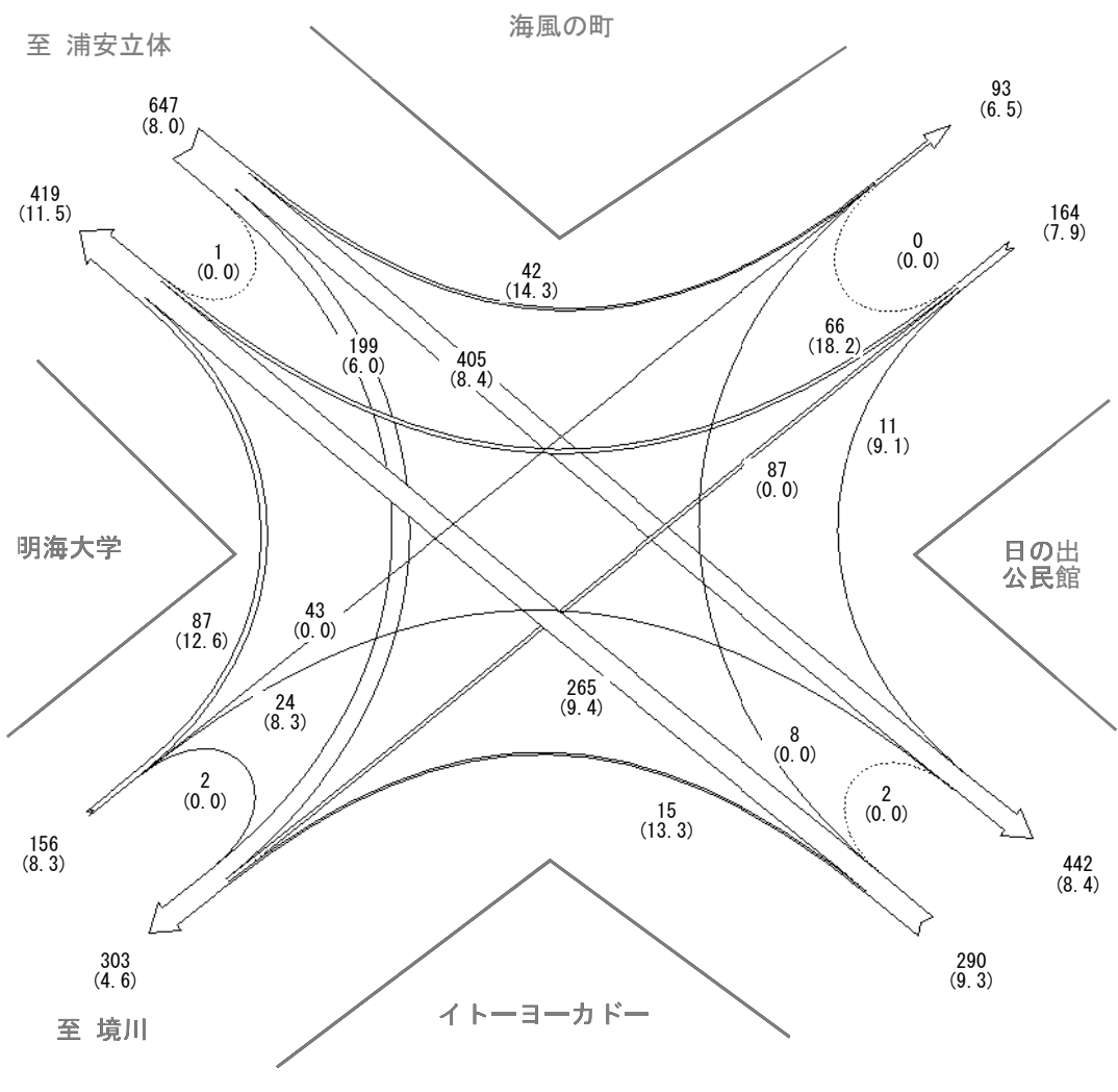
台 / 時間 凡例 50 100 300 ()内は大型車混入率
