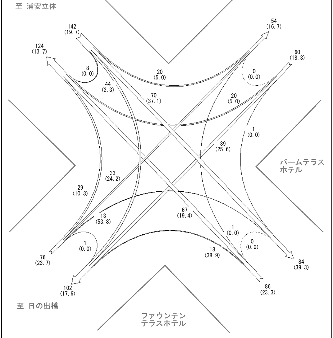
台 / 時間 凡例 20 50 100 () 内は大型車混入率
