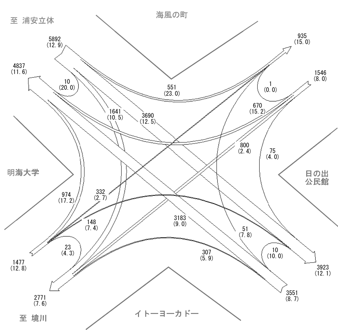
台 / 12 時間 凡例 500 1,000 2,000 ()内は大型車混入率
