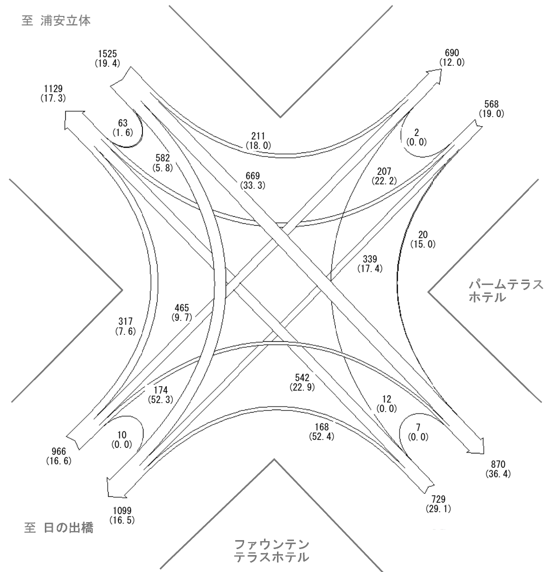
台 / 12 時間 凡例 100 200 500 () 内は大型車混入率
