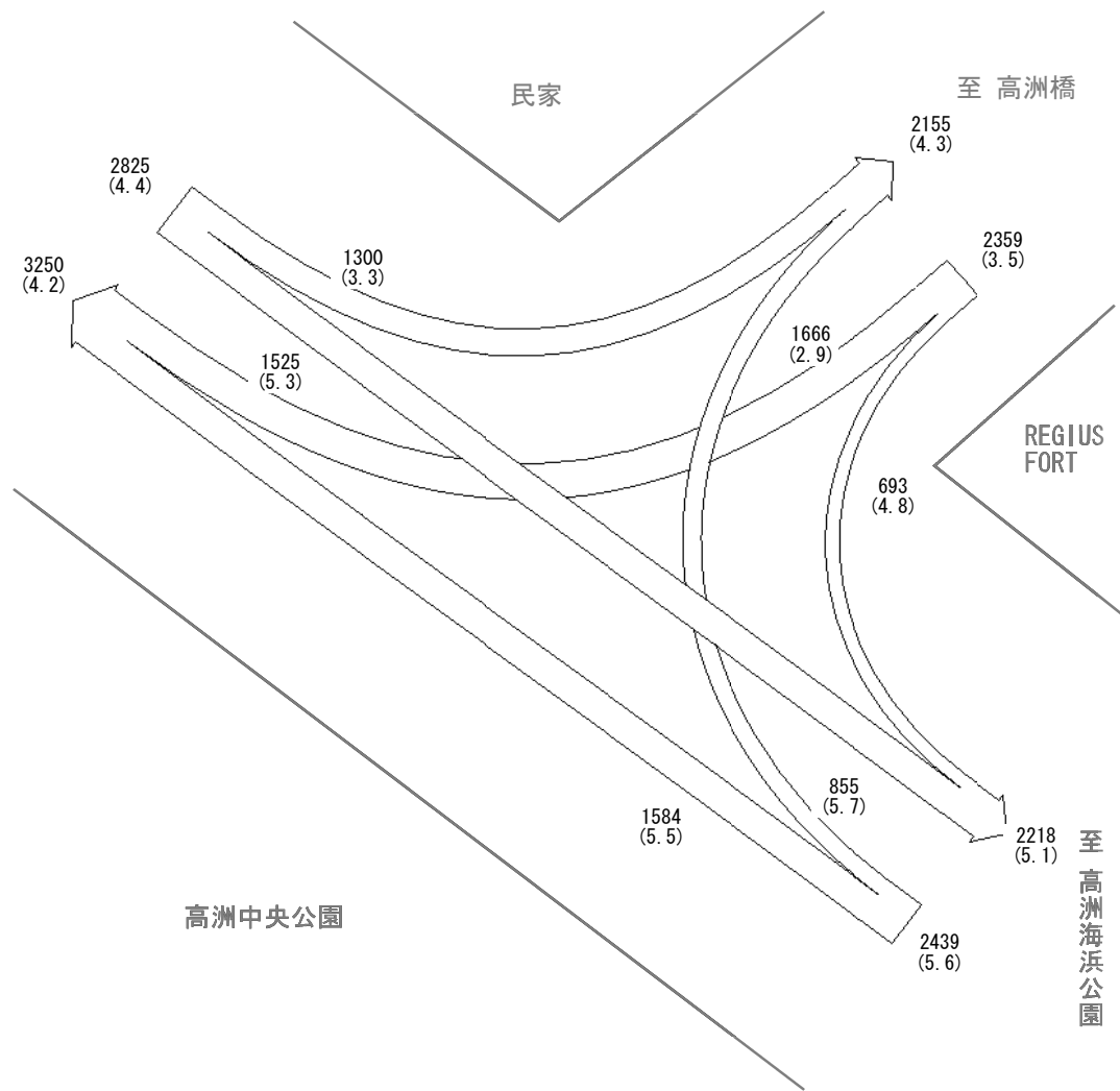
台 / 12 時間 凡例 200 500 1,000 () 内は大型車混入率
