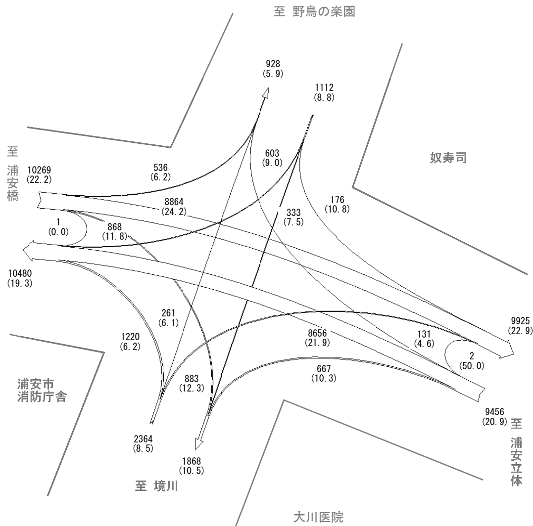
台 / 12 時間 凡例 1,000 2,000 5,000 () 内は大型車混入率
