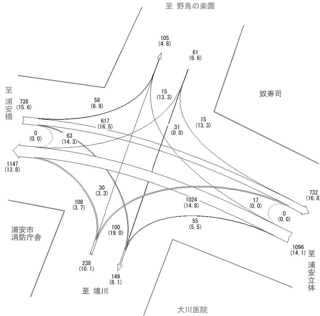
台 / 時間 凡例 100 200 500 () 内は大型車混入率
